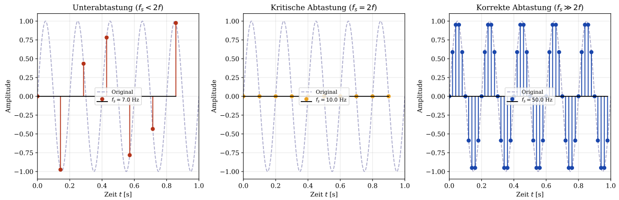
Abbildung 2: Illustration des Nyquist-Shannon-Abtasttheorems (Satz 8) für ein Sinussignal der Frequenz f = 5 Hz. Links: Bei Unterabtastung ( f_s = 7 Hz < 2 \cdot 5 Hz) tritt Aliasing auf; das rekonstruierte Signal würde eine falsche Frequenz zeigen. Mitte: An der Nyquist-Rate ( f_s = 10 Hz) ist eine theoretisch perfekte, aber praktisch empfindliche Rekonstruktion möglich. Rechts: Bei weit überkritischer Abtastung ( f_s = 50 Hz) ist die Hüllkurve des analogen Signals klar erkennbar. In jedem Fall bleibt das analoge Signal die primäre Entität; die Abtastwerte sind Messergebnisse einer diskreten Projektion.
