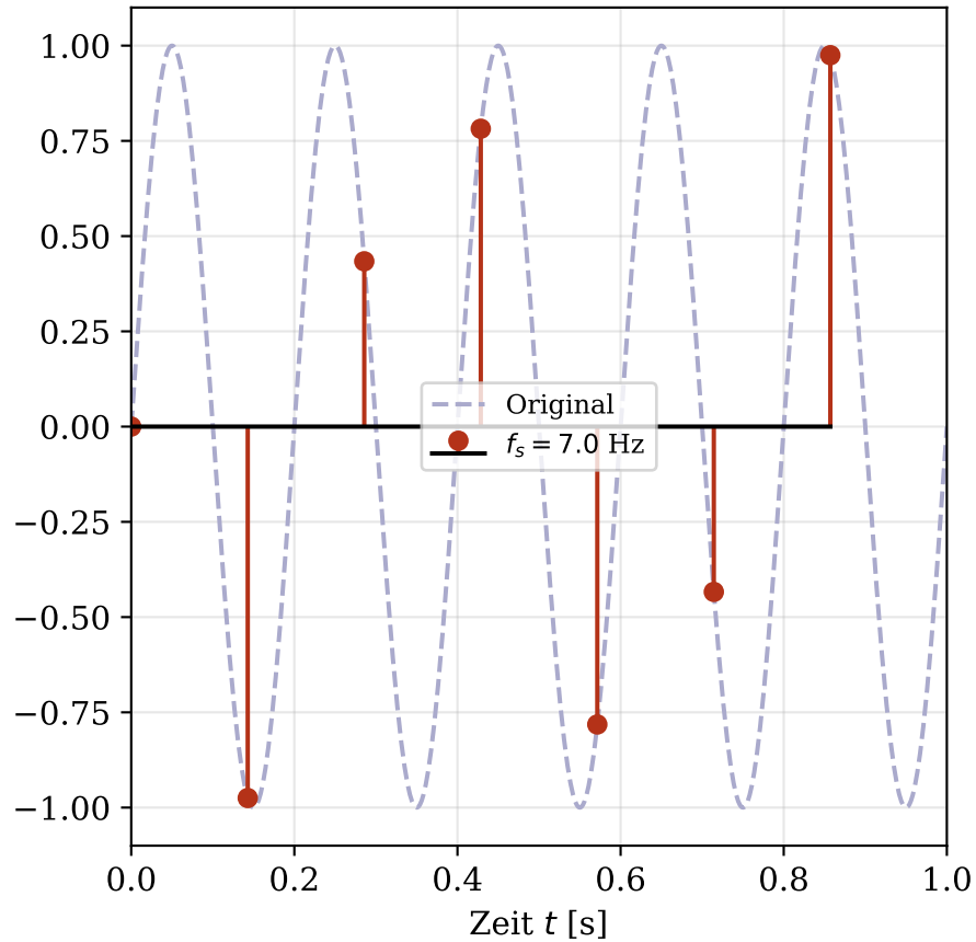
Unterabtastung ( f_s < 2f )
