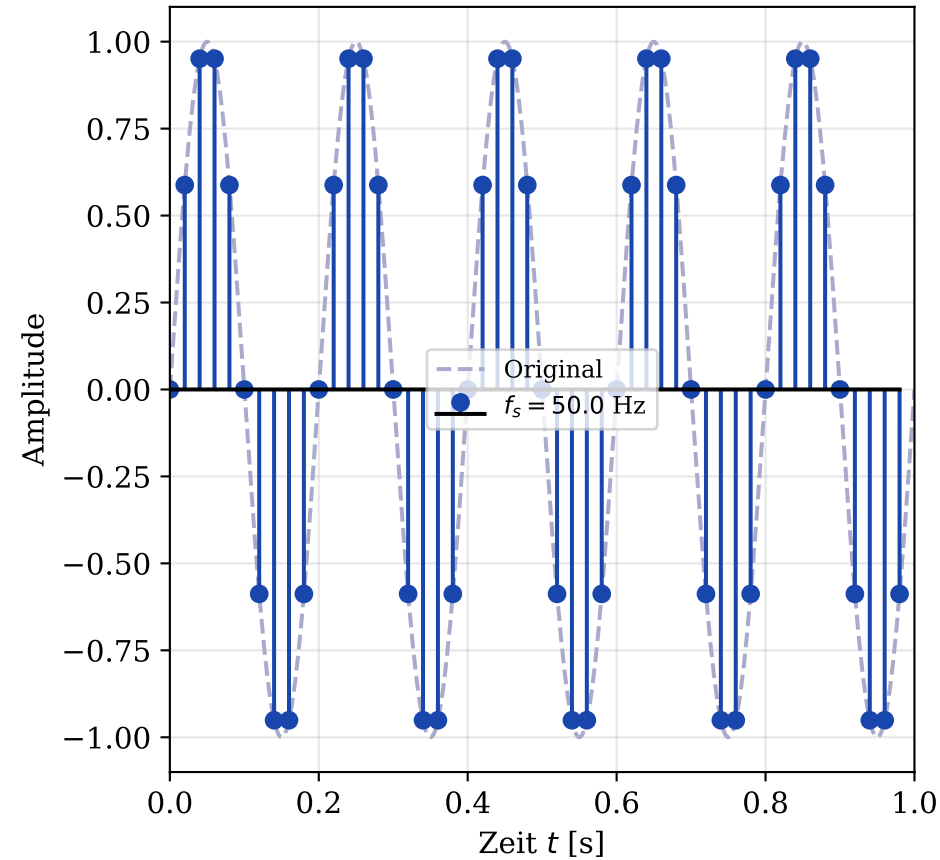
Korrekte Abtastung ( f_s \gg 2f )
