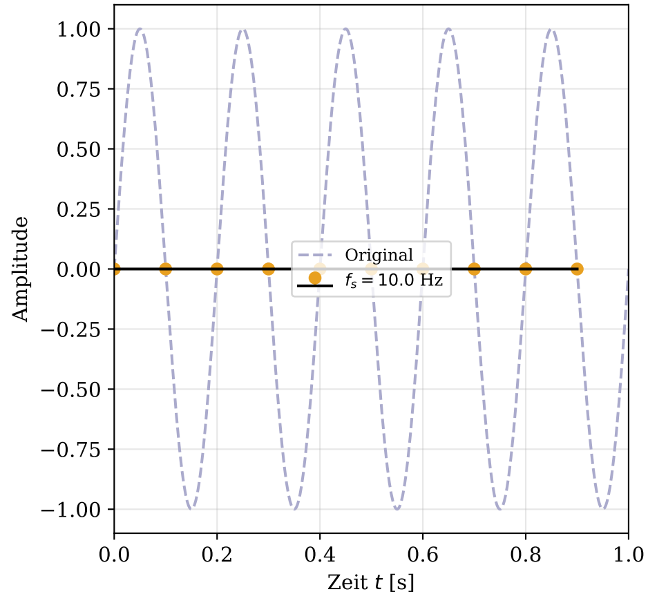
Kritische Abtastung ( f_s = 2f )
