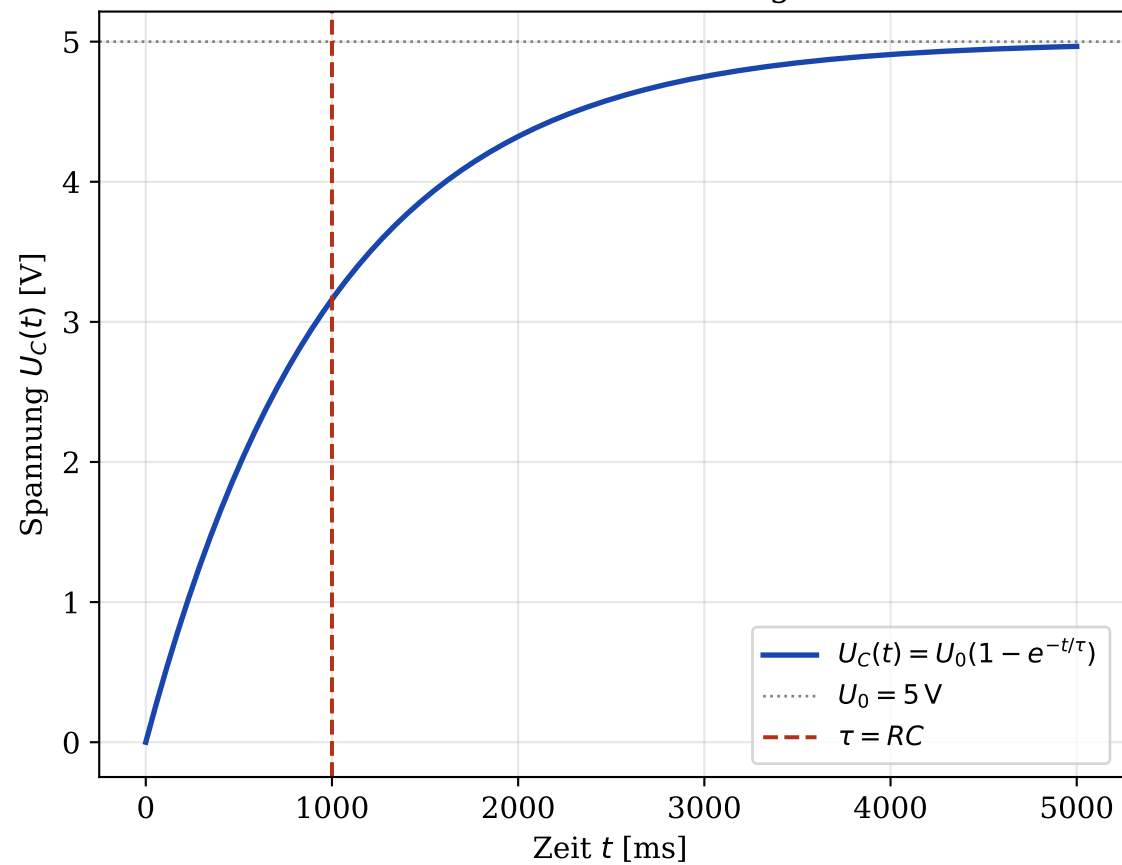
RC-Glied: Aufladung
