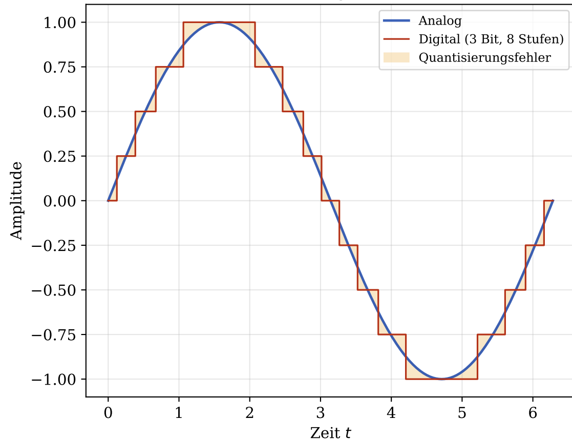
3-Bit-Quantisierung (LSB = 0.2500)
