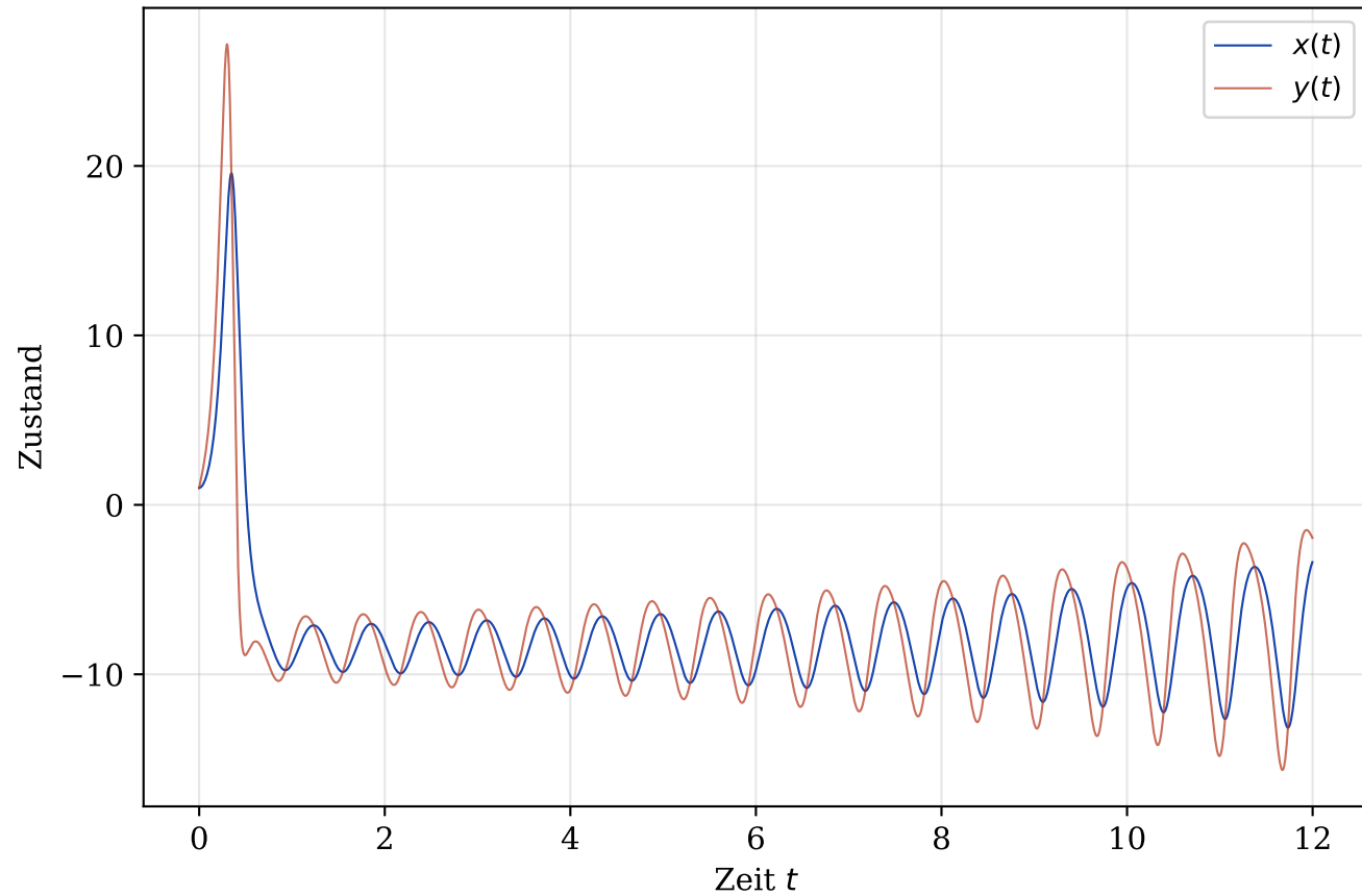
Lorenz: Zeitverlauf
