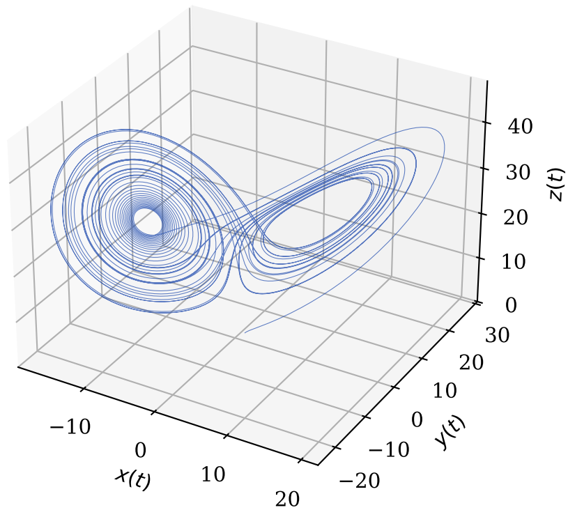
Lorenz-Attraktor (kontinuierlich)
