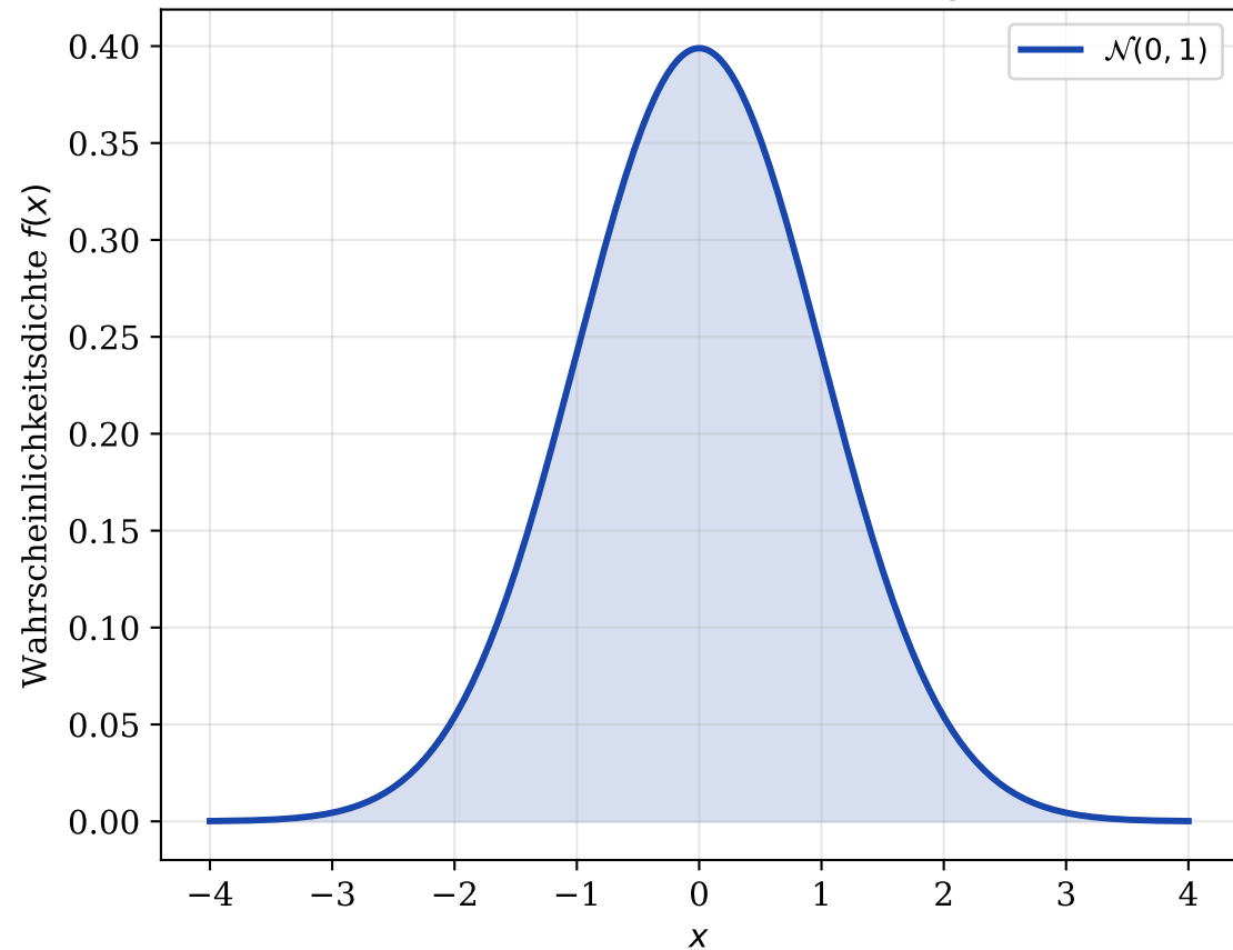
Kontinuierliche Normalverteilung (PDF)
