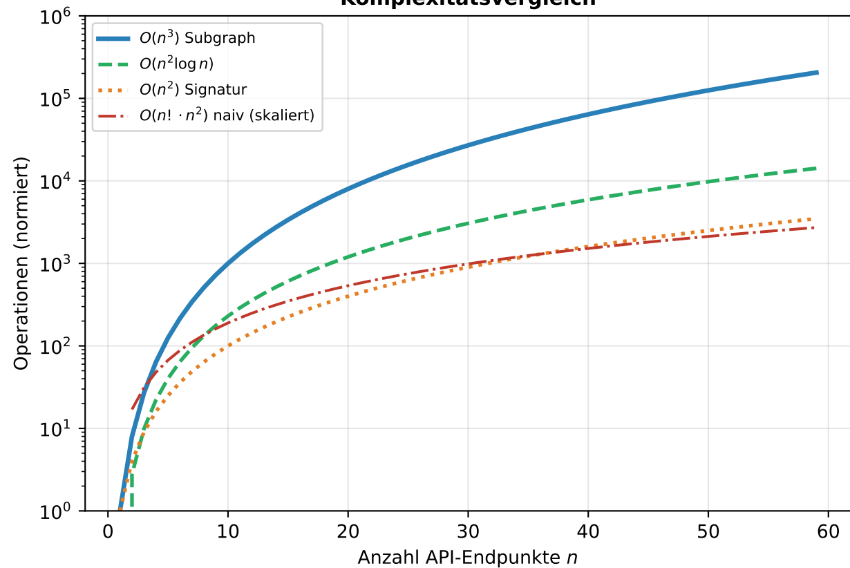
Komplexitätsvergleich
