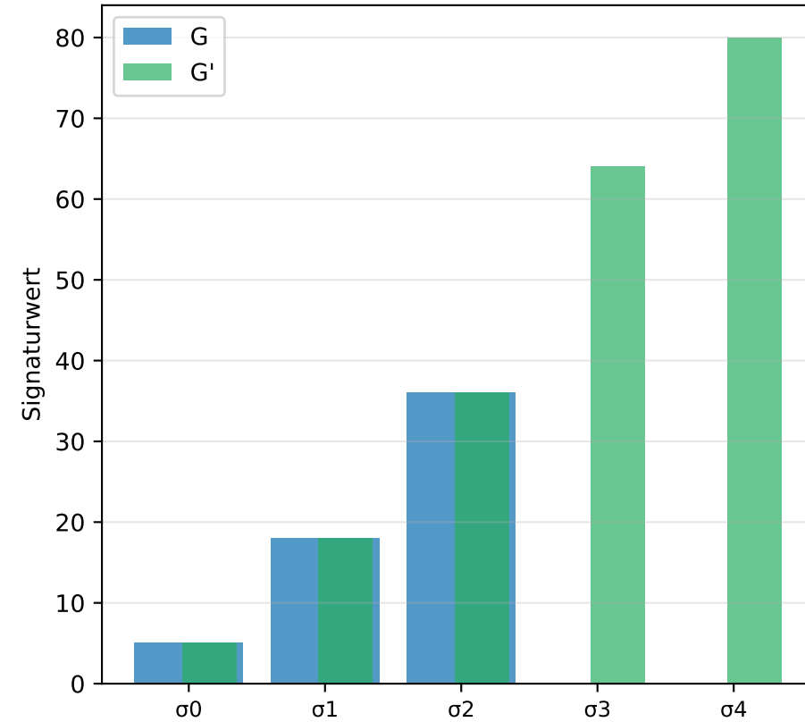
Signatur-Vergleich: G \subseteq G'
