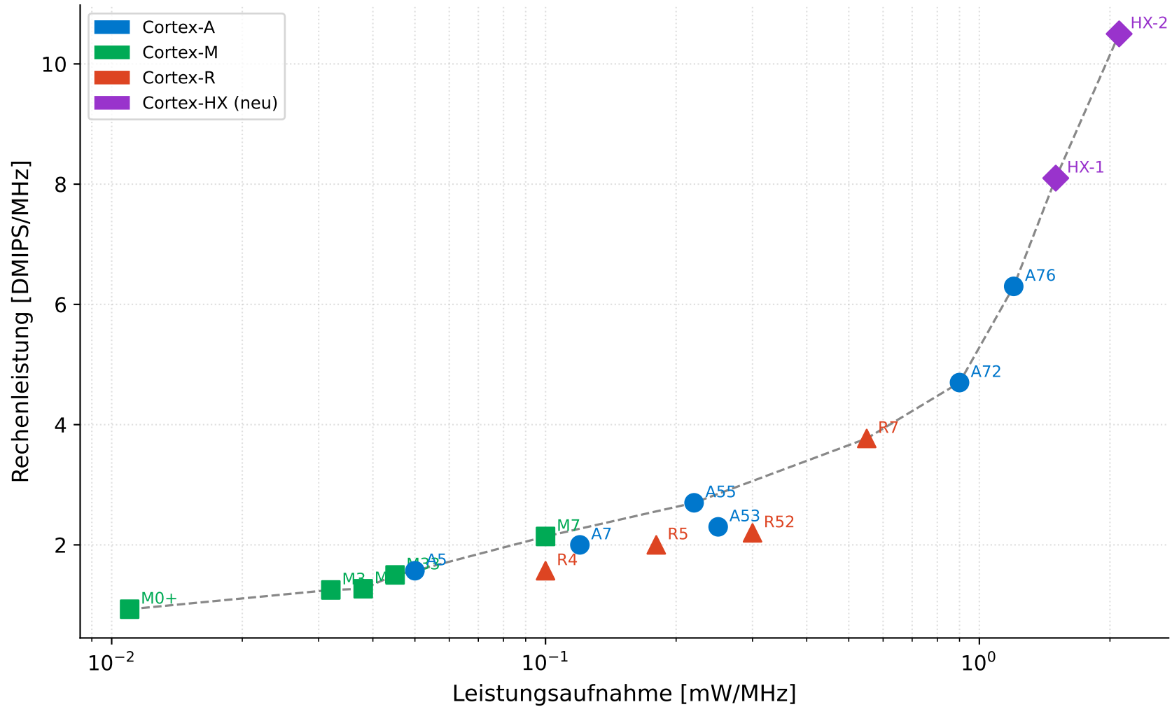
Abb. 1: Performance-Power-Raum der ARM-Cortex-Familien (inkl. neuer HX-Architektur)
