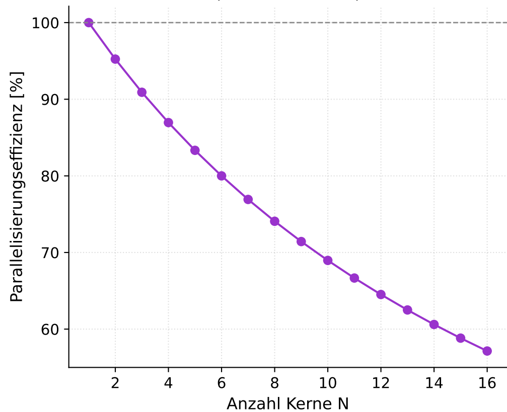
Abb. 6b: Parallelisierungseffizienz (Amdahl-Gesetz)
