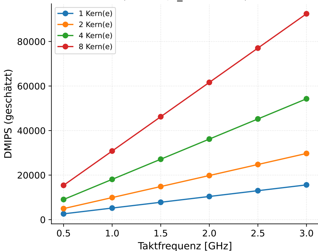
Abb. 6a: Cortex-HX Skalierung (Amdahl, f_{\text{serial}}=0.05 )
