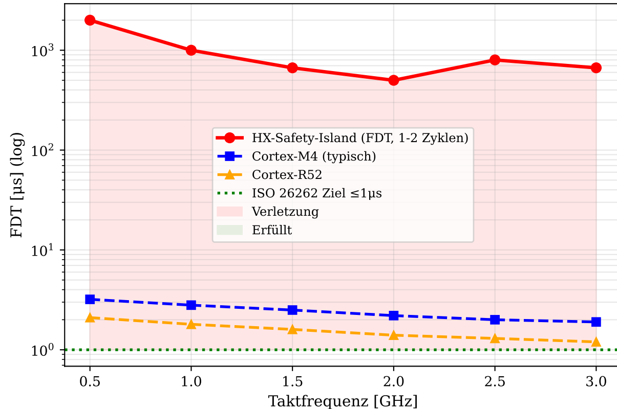
Fehlererkennungszeit vs. Taktfrequenz (ISO 26262 Ziel: FDT ≤ 1µs)
