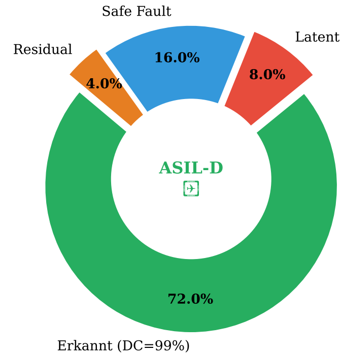
Fehlerverteilung Safety-Island (FMEDA Gesamt - 1847 Fehlermoden)
