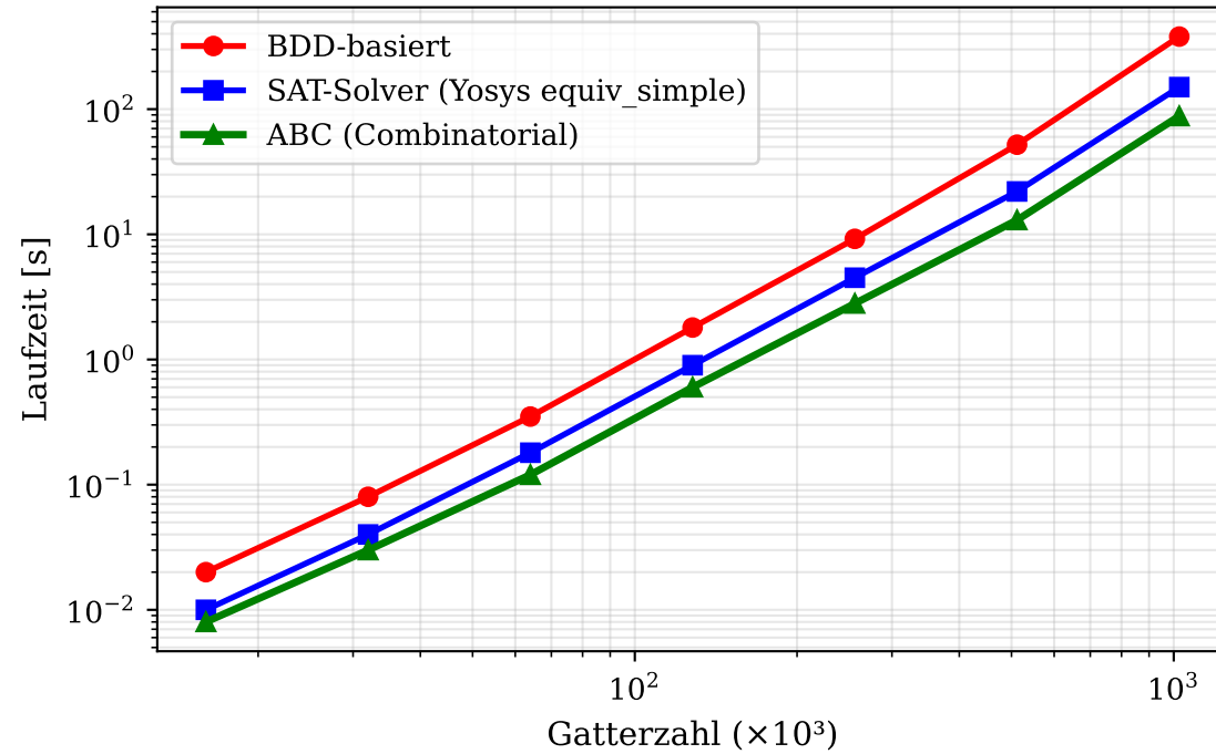
Äquivalenzprüfungs-Laufzeit vs. Schaltungsgröße
