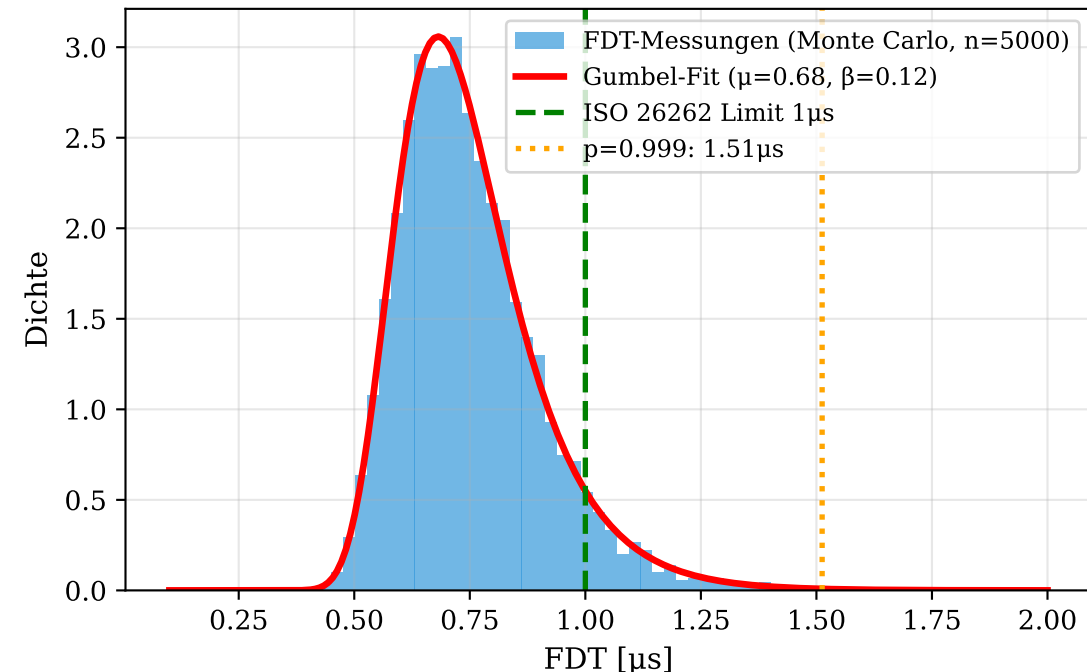
FDT-Verteilung (Monte Carlo Simulation) Safety-Island @2GHz
