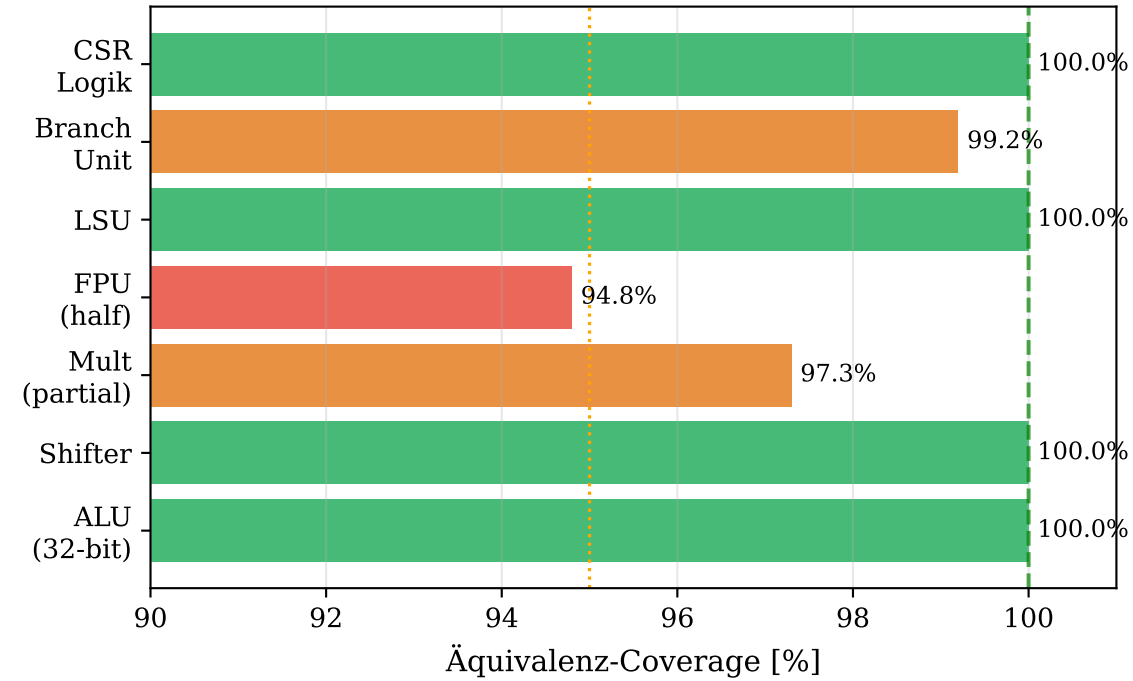
Coverage-Ergebnis je Modul (Yosys equiv_check)
