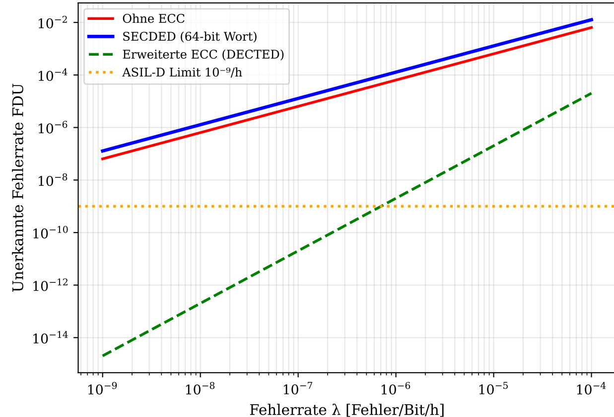
Unerkannte Fehlerrate FDU vs. Einzel-Fehlerrate \lambda
