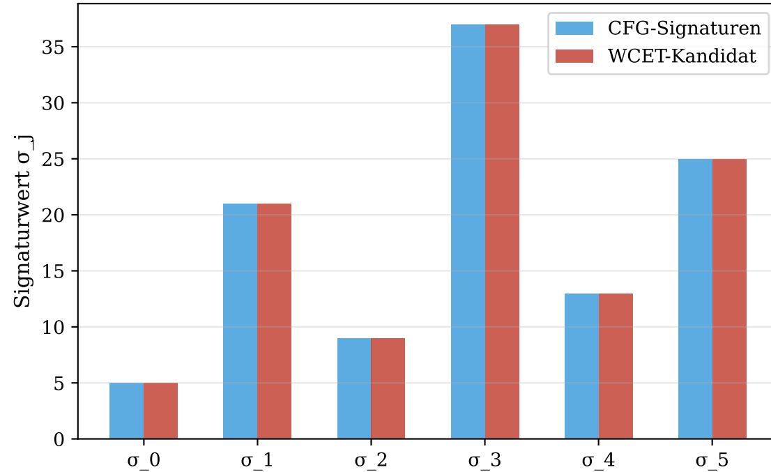
Signaturvergleich CFG vs. WCET-Kandidat
