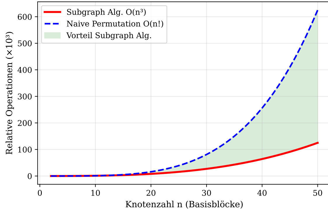
Komplexitätsvergleich: O(n^3) vs. O(n!)
