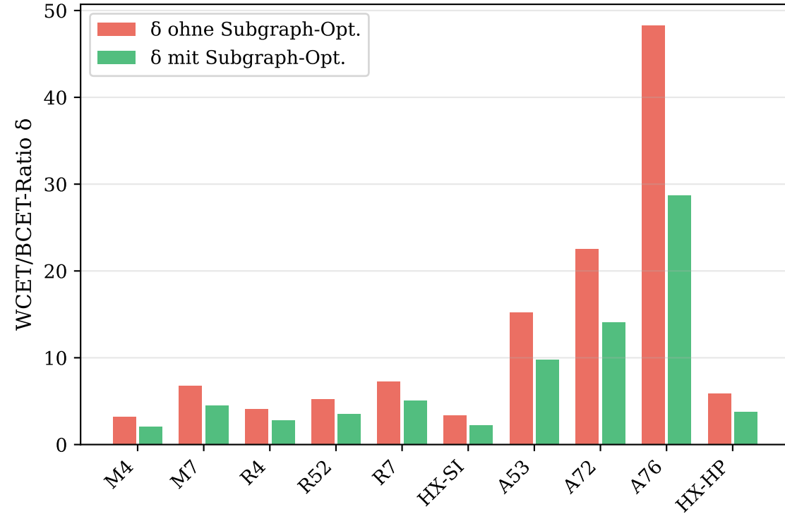
Reduktion des WCET-Spreads \delta durch Subgraph-Analyse
