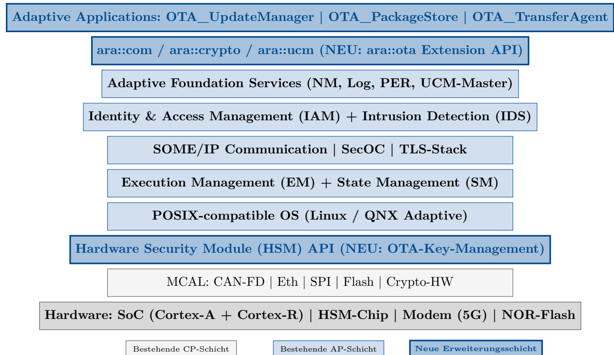
Abbildung 9: Erweitertes AUTOSAR-Schichtenmodell für das ZSG. Neue Schichten und Dienste sind blau hervorgehoben. Der OTA-Manager ist als Adaptive Application implementiert.
