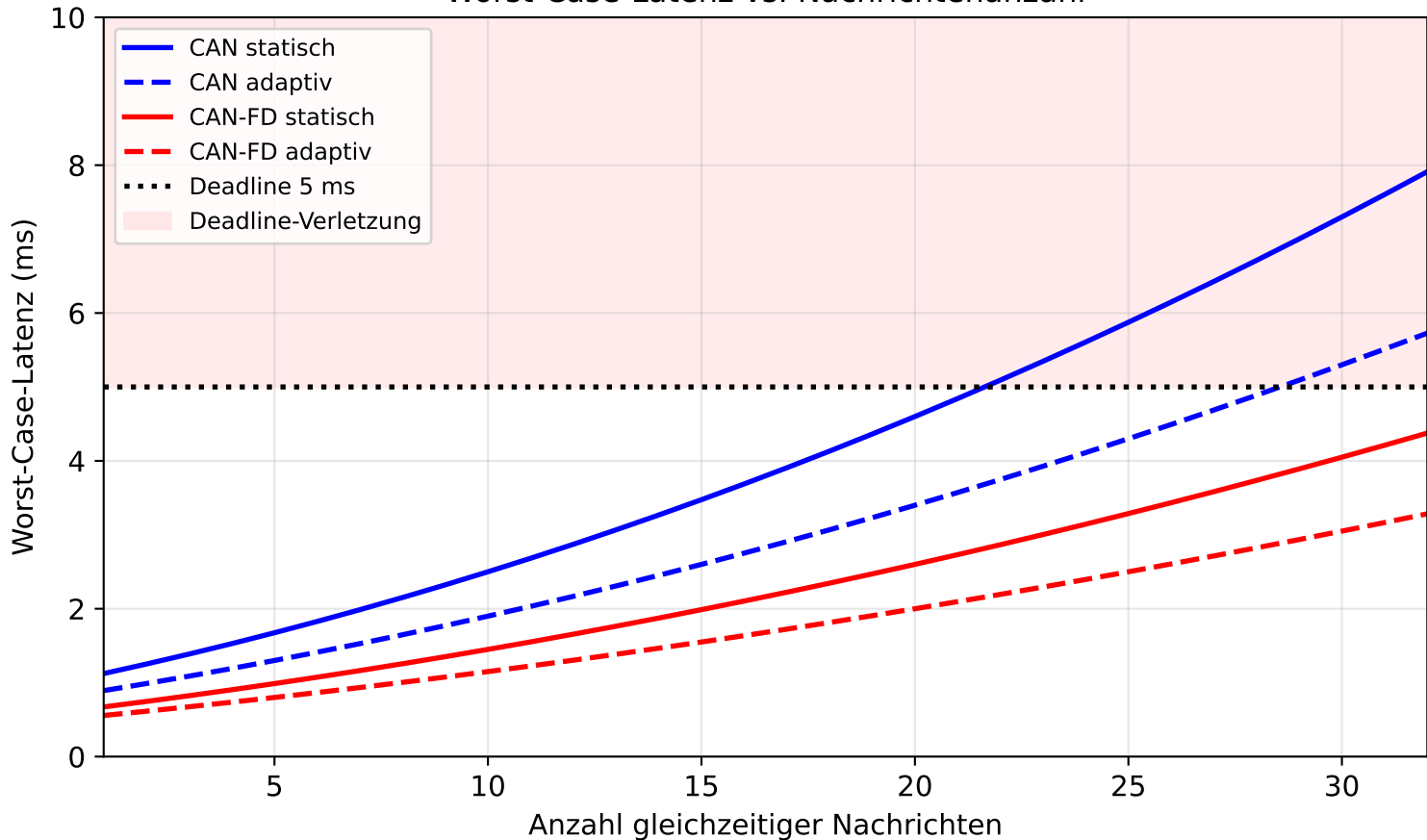
Worst-Case-Latenz vs. Nachrichtenanzahl
