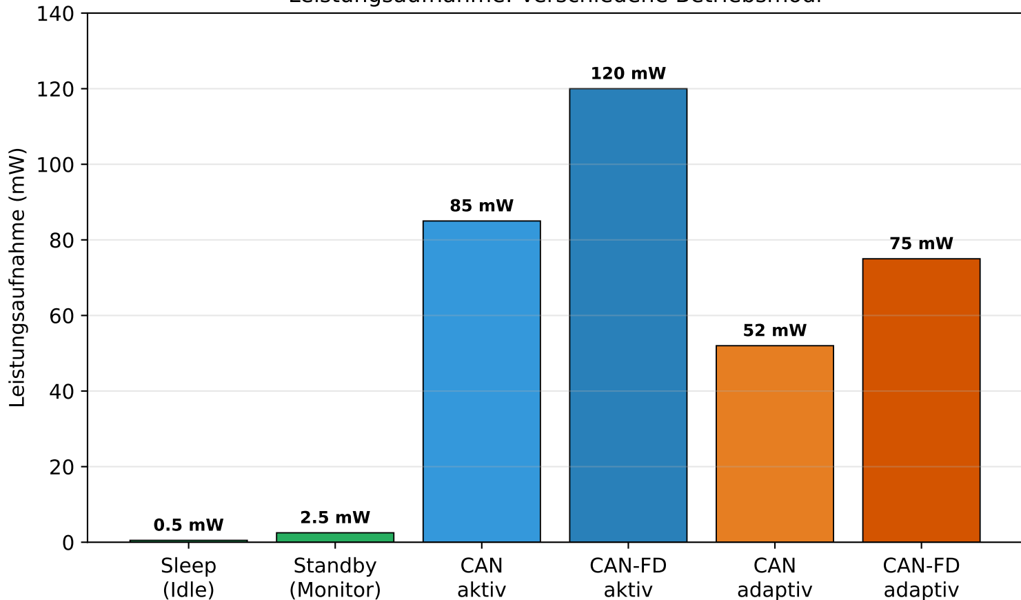
Leistungsaufnahme: Verschiedene Betriebsmodi
