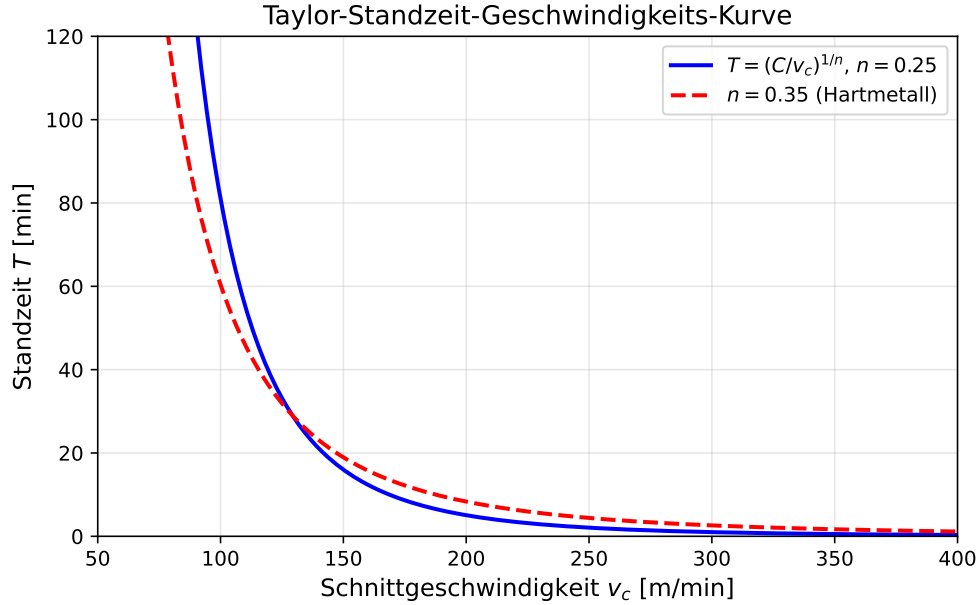
Abbildung 1: Taylor-Standardzeit-Geschwindigkeits-Kurven für zwei Schneidstoffklassen (Taylor-Exponent n = 0,25 für HSS/Standardhartmetall, n = 0,35 für beschichtetes Hartmetall). Mit steigendem Taylor-Exponenten wird die Kurve flacher, was eine größere Werkzeugbandbreite bezüglich v_c bedeutet.
