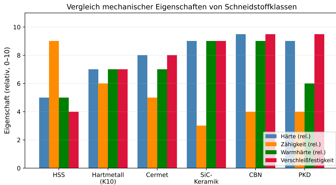
Abbildung 5: Relativer Vergleich mechanischer Kenngrößen verschiedener Schneidstoffklassen (Skala 0–10, normiert). PKD und CBN dominieren bei Härte und Verschleißfestigkeit; HSS bietet die höchste Zähigkeit und ist damit am unempfindlichsten gegenüber Unterbrechungsschnitten.
