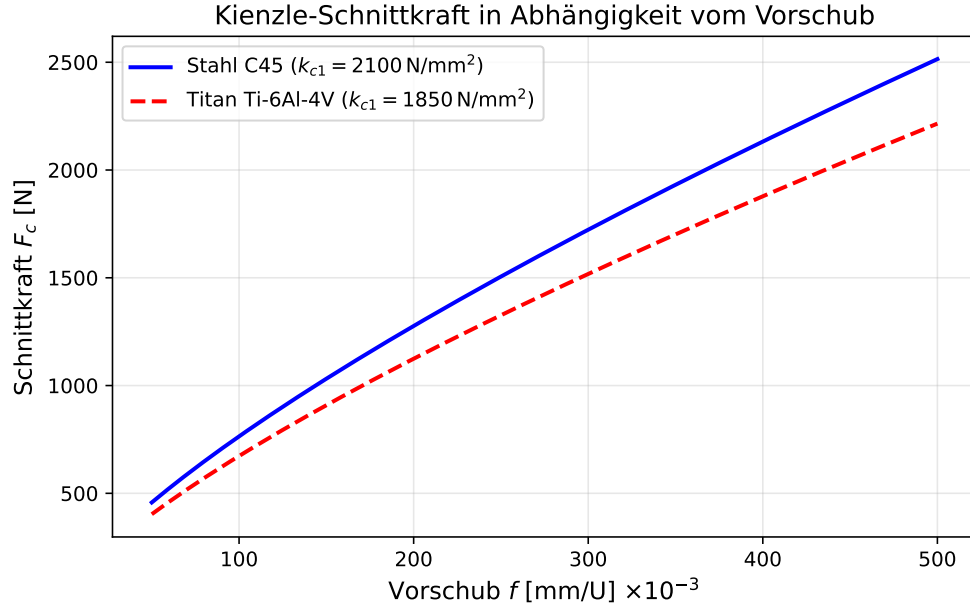
Abbildung 3: Schnittkraft F_c nach dem Kienzle-Modell in Abhängigkeit vom Vorschub f für Stahl C45 ( k_{c1} = 2100 \text{ N/mm}^2 , m_c = 0,26 ) und Titan Ti-6Al-4V ( k_{c1} = 1850 \text{ N/mm}^2 , m_c = 0,26 ), jeweils bei a_p = 2,0 \text{ mm} .
