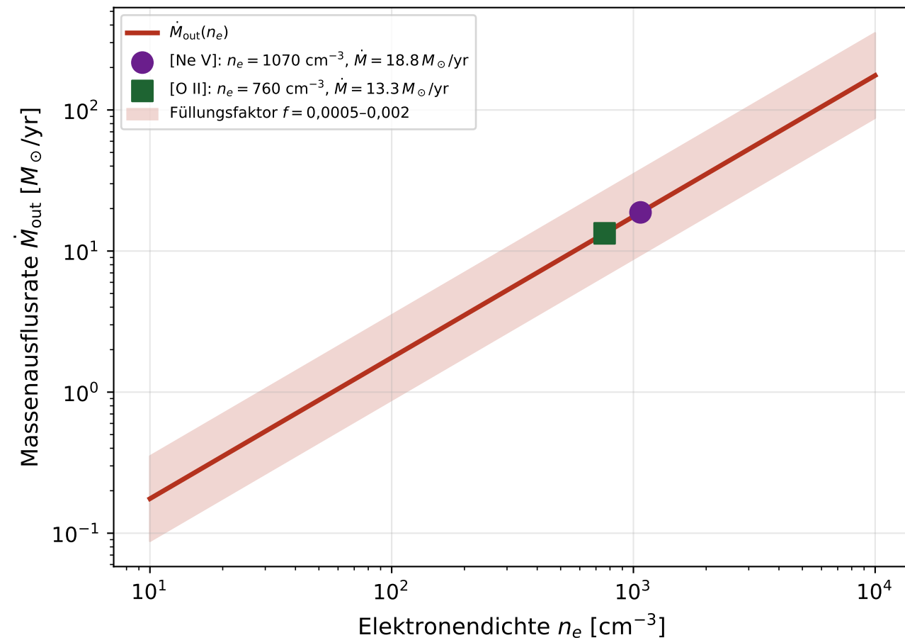
Massenausflusrate vs. Elektronendichte
