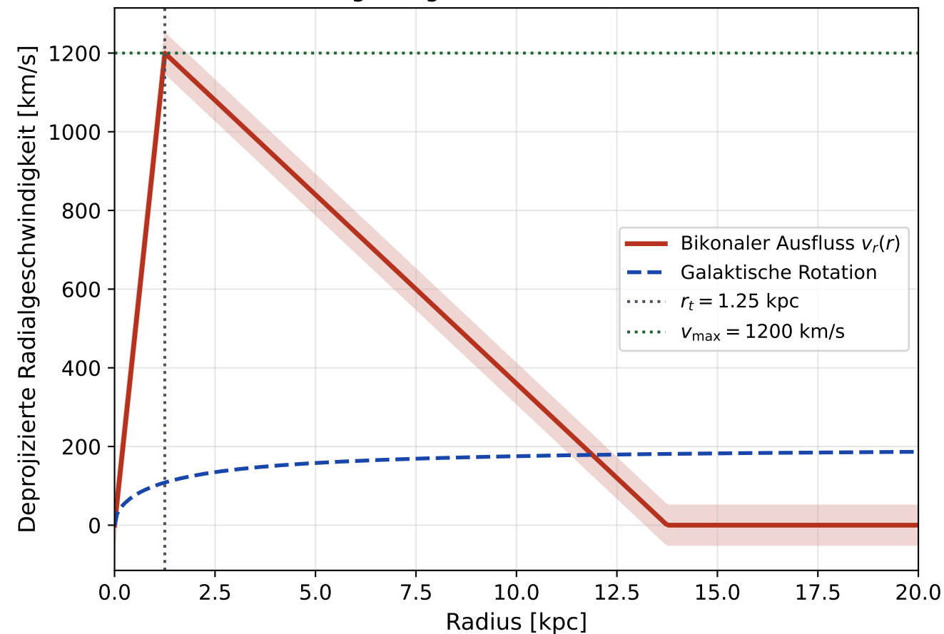
Geschwindigkeitsgesetz des bikonalen Ausflusses
