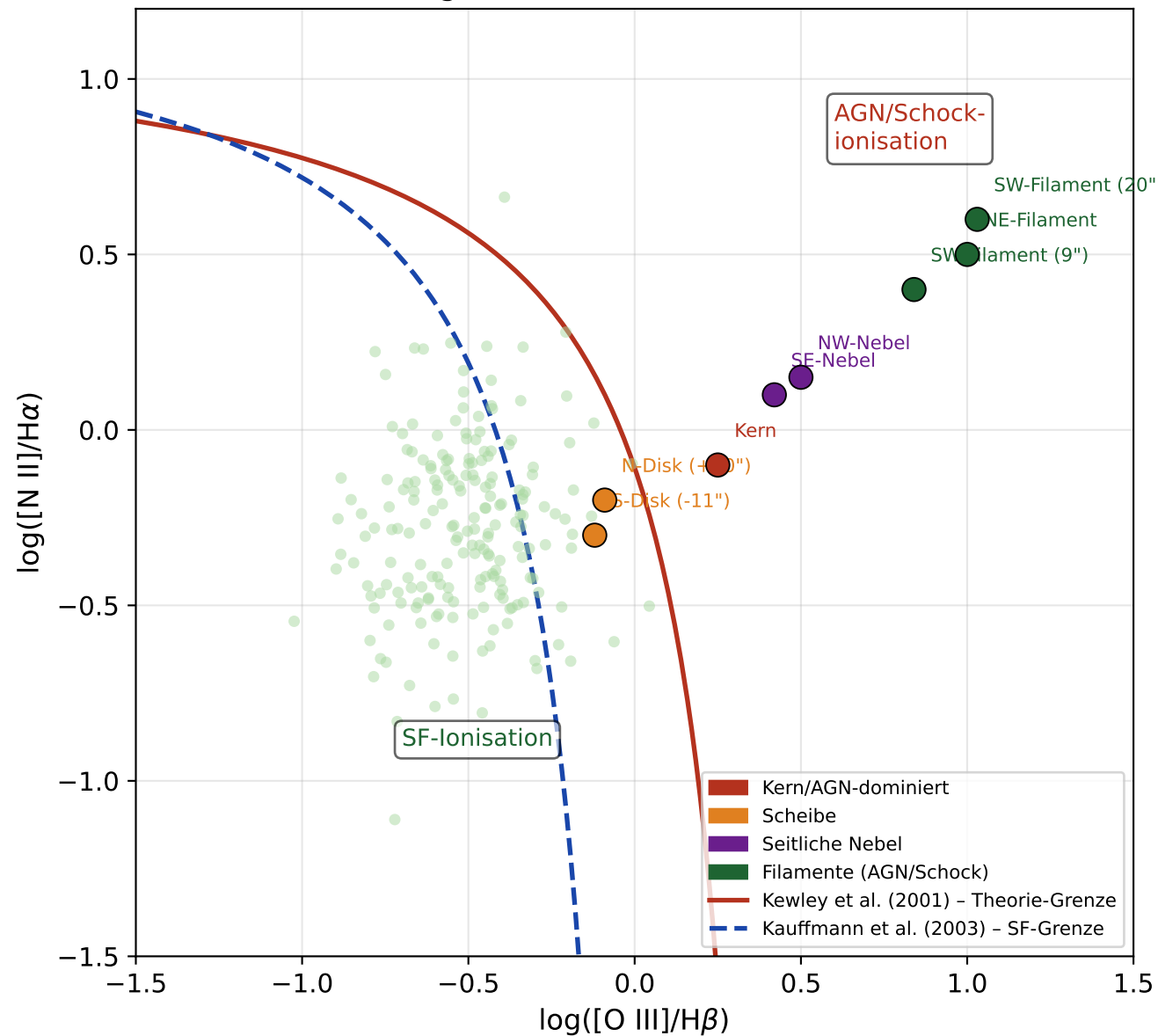
BPT-Diagramm: Ionisationsmechanismen
