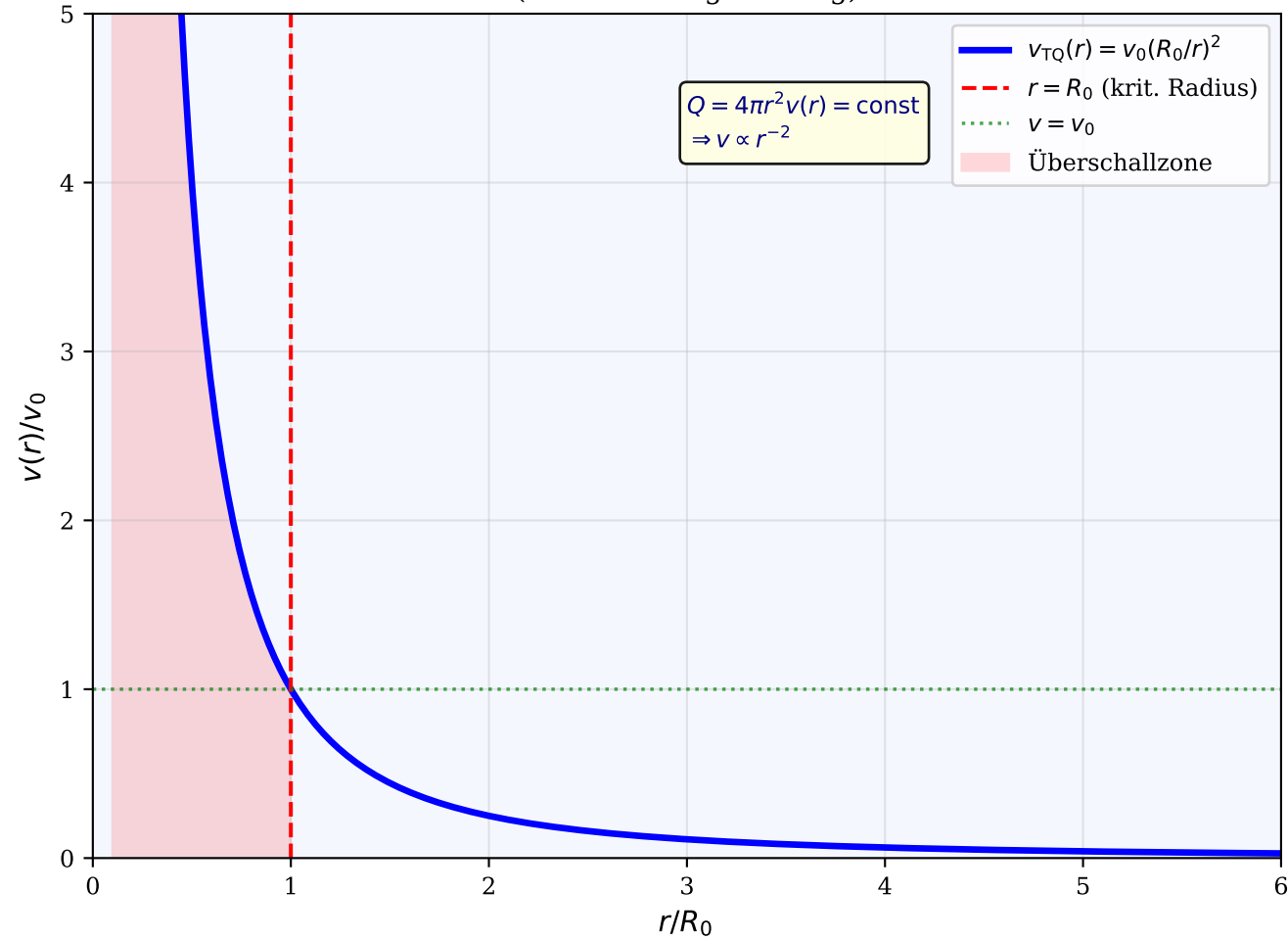
Tiefenquelle: Soggeschwindigkeit (Kontinuitätsgleichung)
