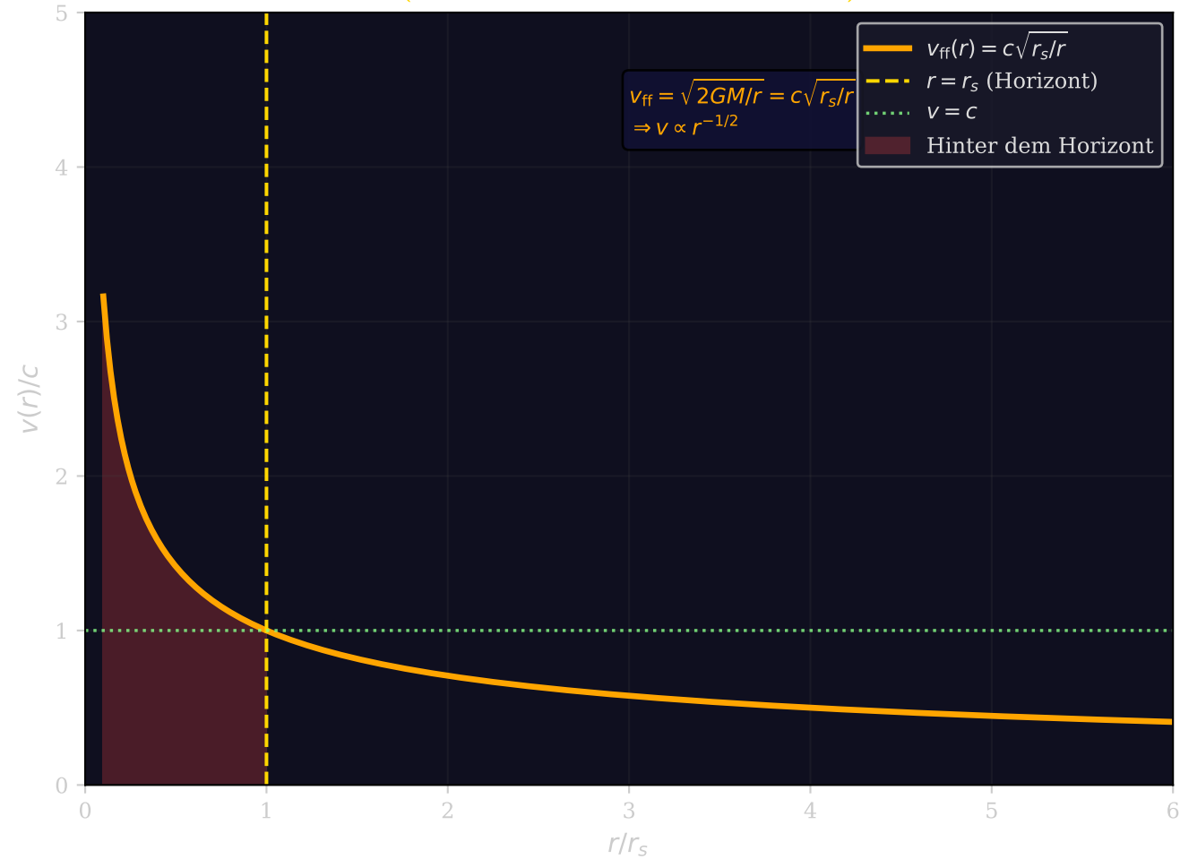
Schwarzes Loch: Freifallgeschwindigkeit (Painlevé-Gullstrand-Koordinaten)
