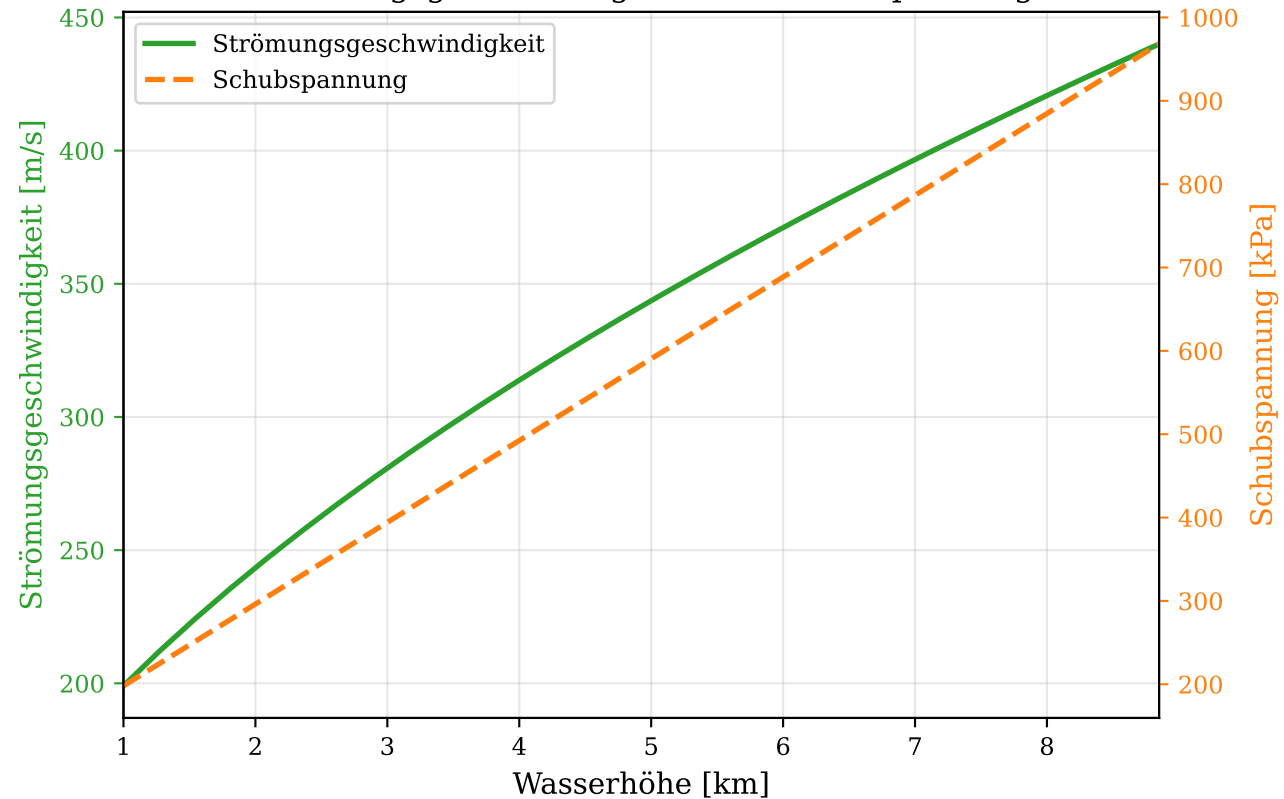
Strömungsgeschwindigkeit und Schubspannung
