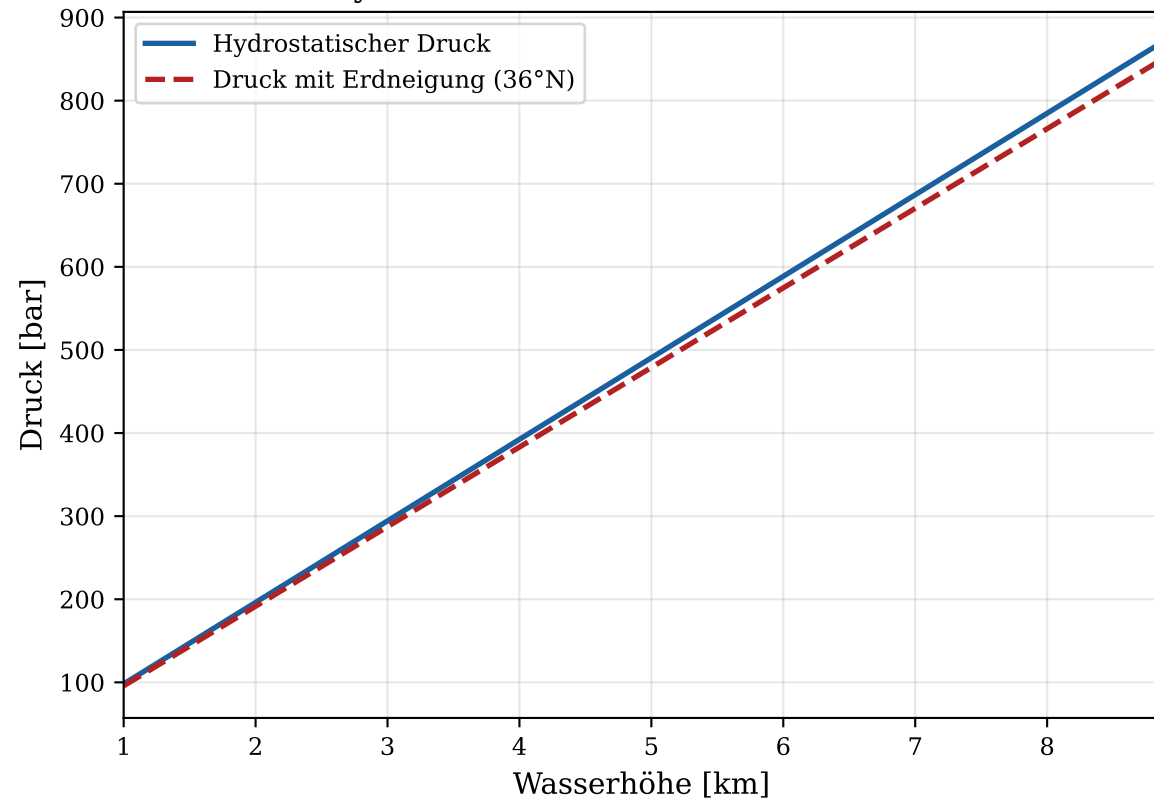
Hydrostatischer Druck vs. Wasserhöhe
