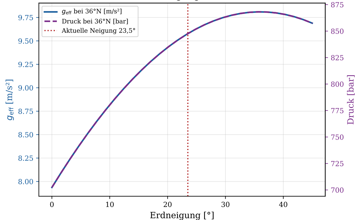
Effektive Gravitation und Druck bei 36°N vs. Erdneigungswinkel
