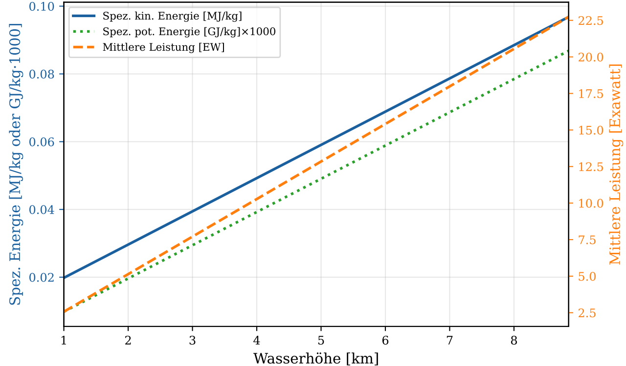
Spezifische Energiedichten und Leistung
