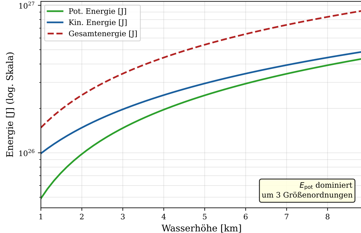
Energieformen vs. Wasserhöhe (logarithmische Skala)
