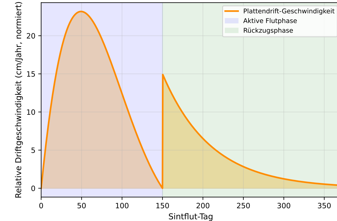
Plattenbewegungsgeschwindigkeit während der Sintflut
