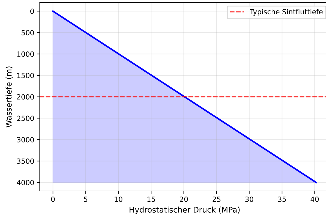
Sintflut: Druckzunahme mit Tiefe
