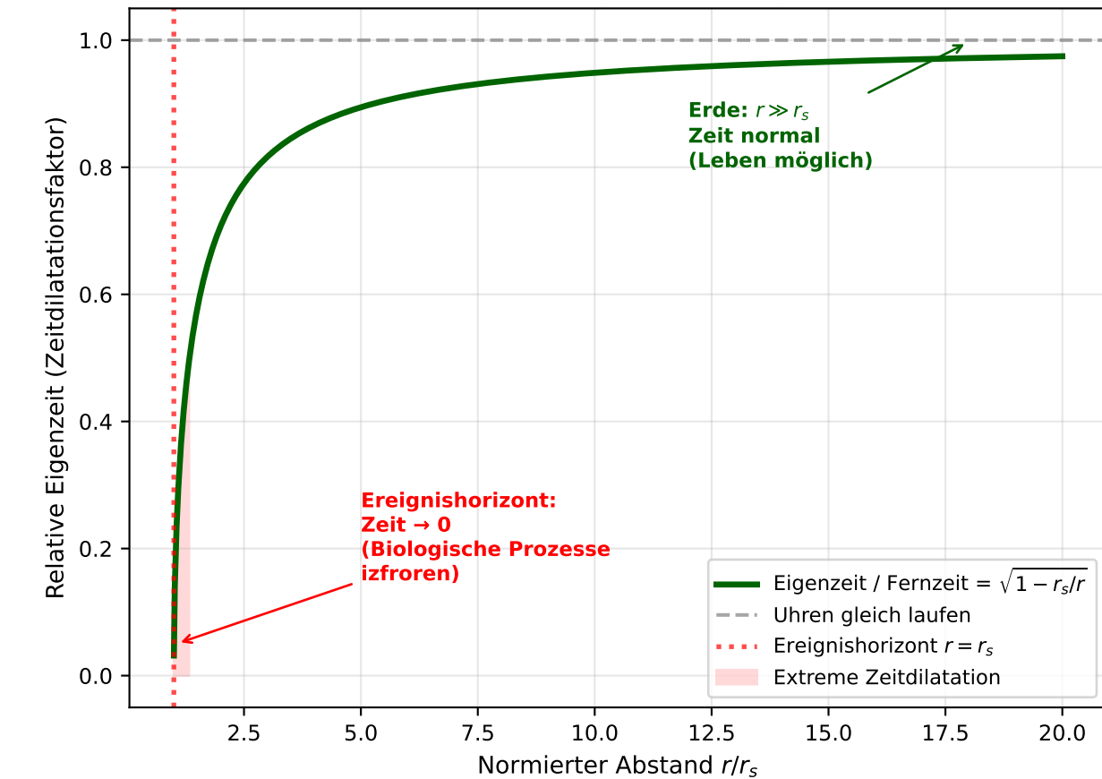
Gravitationszeitdilatation: Zeit kommt zum Erliegen am Ereignishorizont
