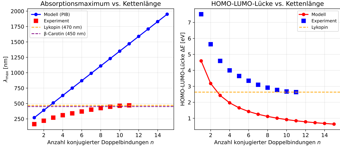
Abbildung 2: Links: Absorptionswellenlänge \lambda_{\max} als Funktion der Zahl konjugierter Doppelbindungen p , verglichen mit experimentellen Werten (Quadrate). Rechts: HOMO-LUMO-Lücke \Delta E in eV. Die gestrichelten Linien markieren die Werte für Lykopen ( p = 11 , \lambda \approx 470 nm, \Delta E \approx 2.64 eV) und \beta -Carotin ( \lambda \approx 450 nm).
