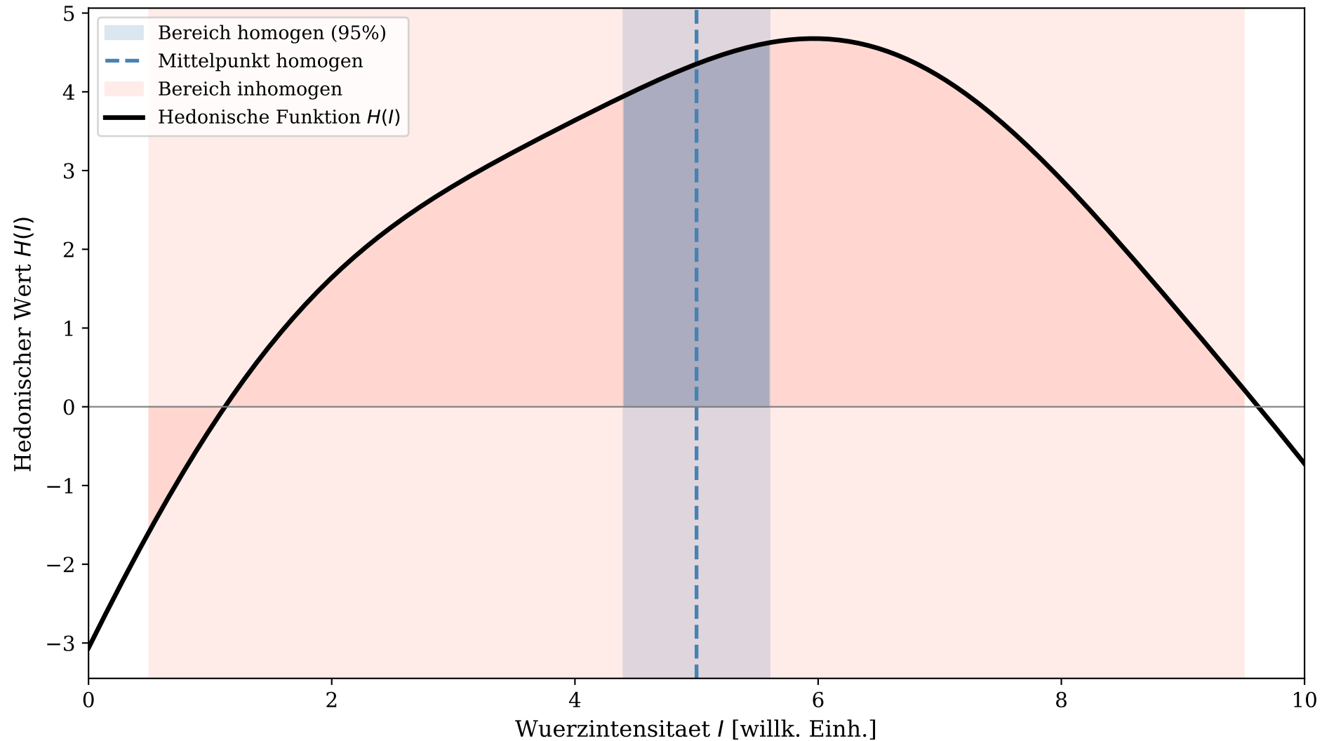
Abb. 2: Wundt-Kurve der Geschmacksreaktion mit Stimulationsbereichen
