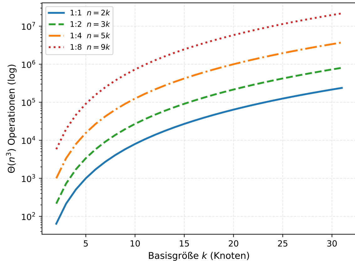
Subgraph-Isomorphismus-Komplexität nach CPU:GPU-Konfiguration
