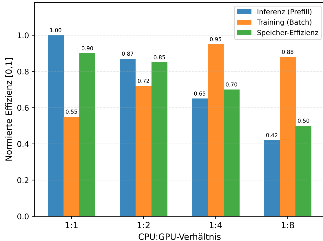
Workload-spezifische Effizienz nach CPU:GPU-Konfiguration
