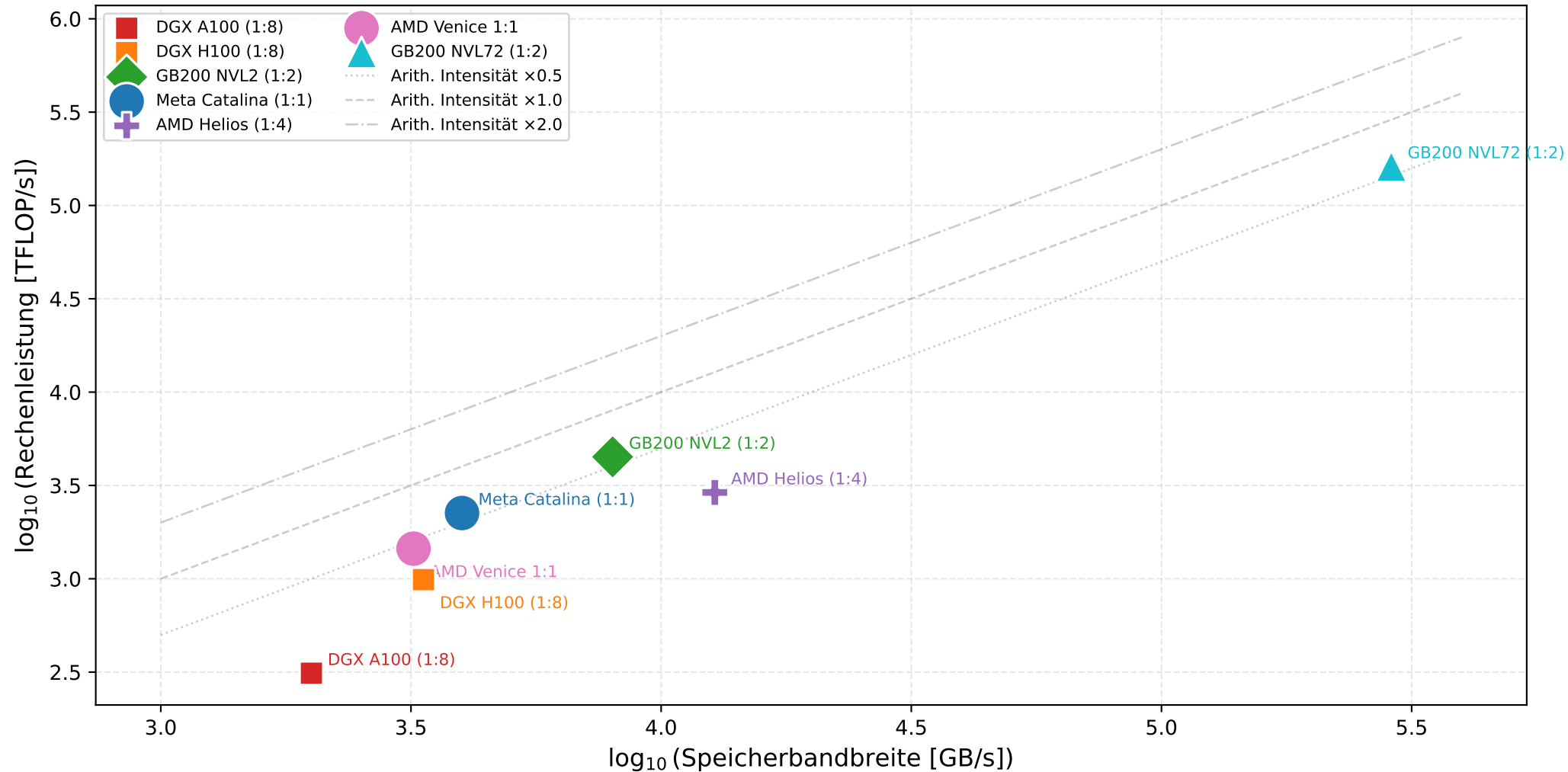
Abbildung 3: Speicherbandbreite vs. Rechenleistung nach Plattform und CPU:GPU-Verhältnis
