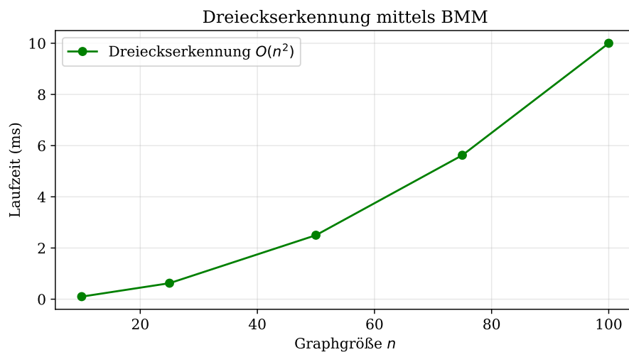
Abbildung 2.8: Dreieckserkennung mittels BMM. Die Laufzeit wächst quadratisch mit der Graphgrösse.
