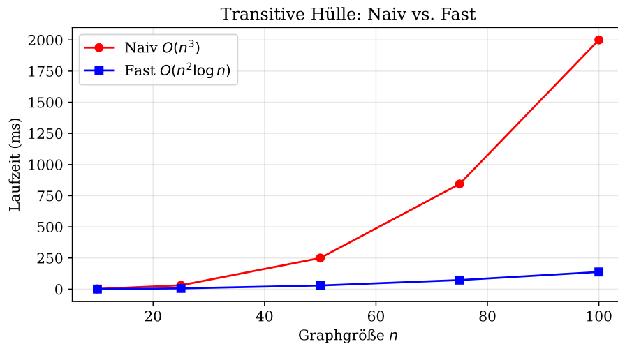
Abbildung 2.7: Vergleich der Transitive-Hülle-Algorithmen. Das wiederholte Quadrieren (Fast) ist deutlich schneller als die naive Methode für grössere Graphen.
