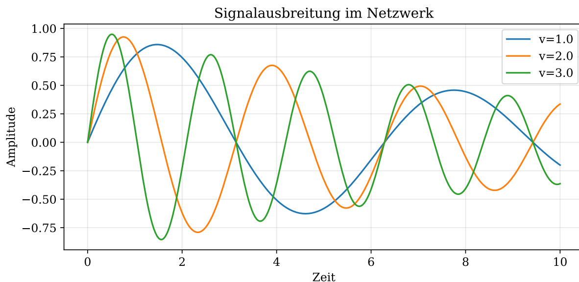
Abbildung 14.7: Netzwerke: Signalausbreitung und Spektralradius
