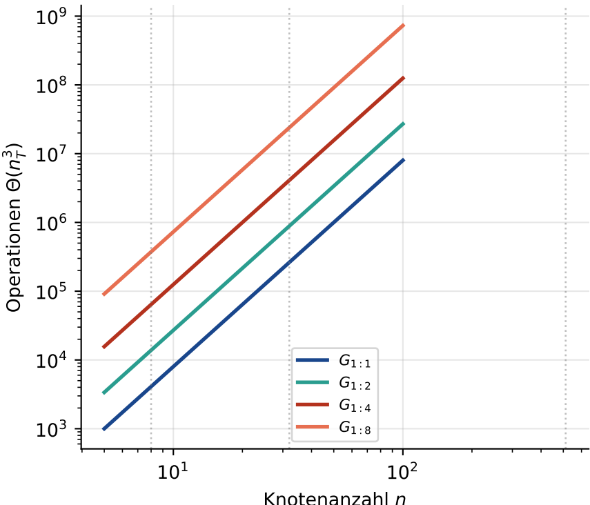
Subgraph Algorithmus Komplexität nach CPU:GPU-Konfiguration
