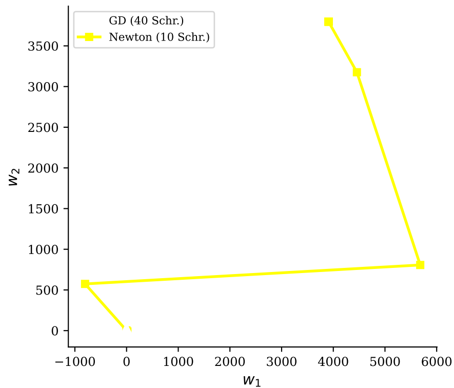
Geodätiken auf \mathcal{M} : GD vs. Newton
