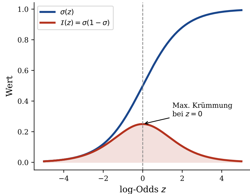
Fisher-Information der Bernoulli-Verteilung (Depensions-Krümmung)
