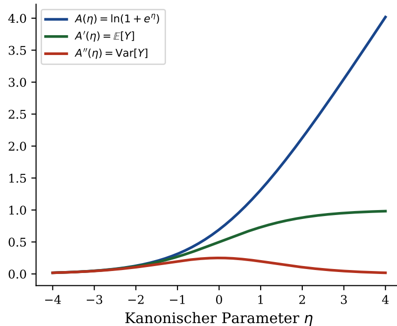
Log-Partition-Funktion und Momente der Depension
