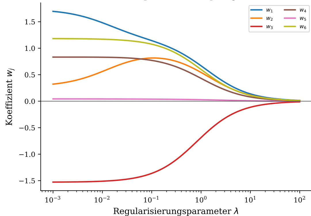
Ridge-Regularisierungspfad (L2-Depensions-Dämpfung)
