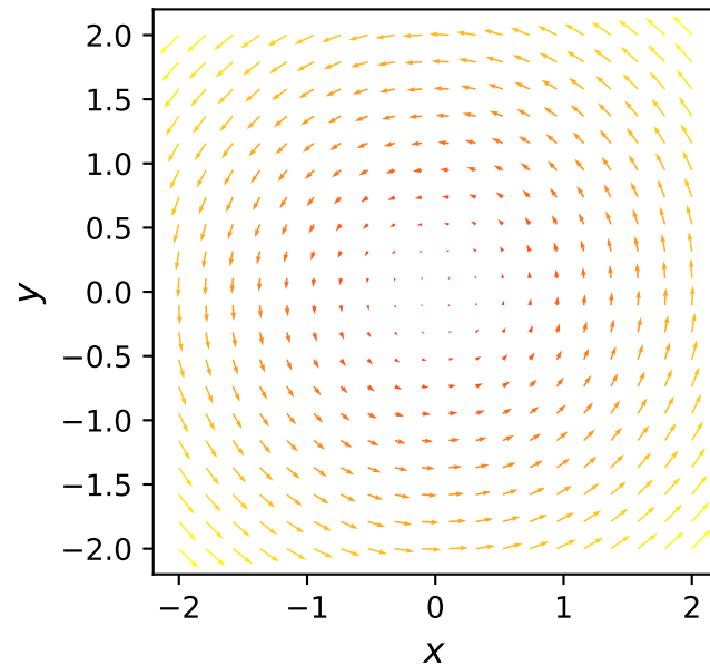
Quiver-Plot (Vektorfeld)
