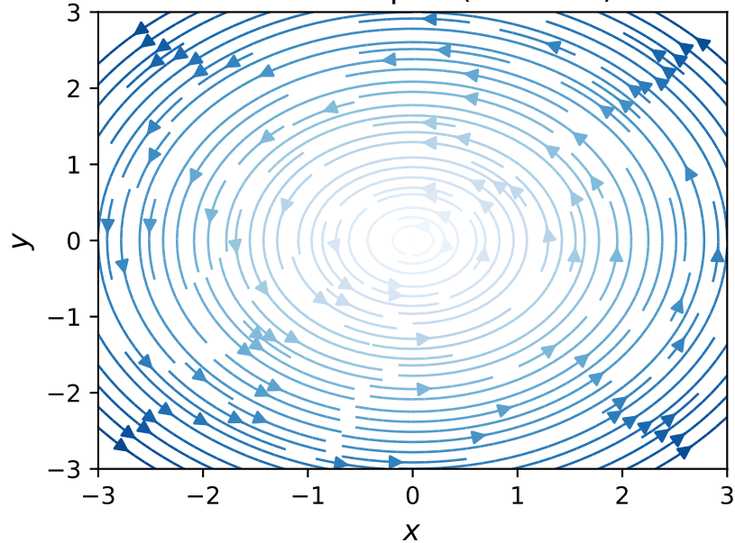
Stromlinienplot (Rotation)
