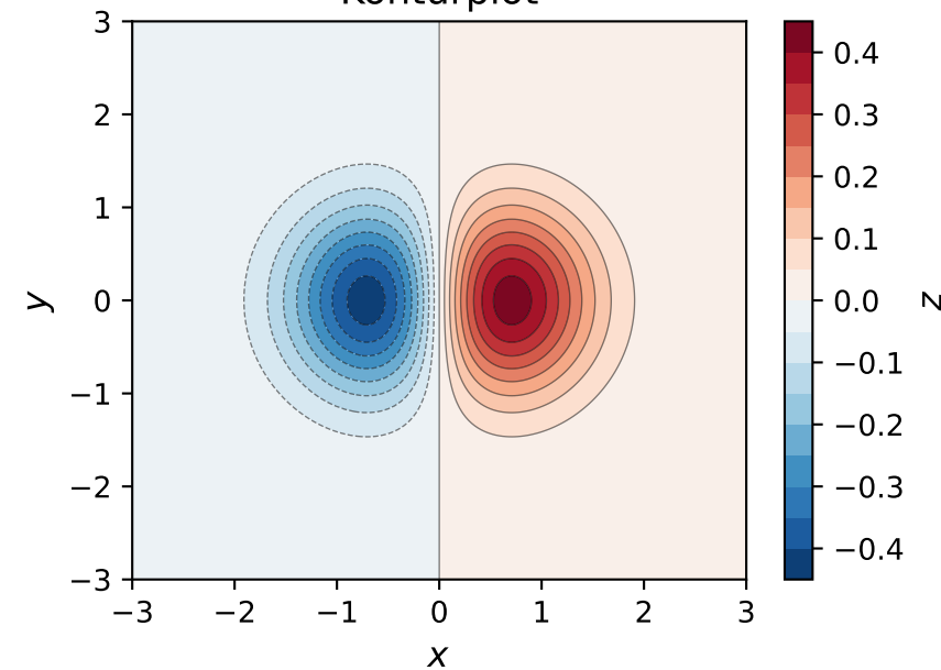
Konturplot
