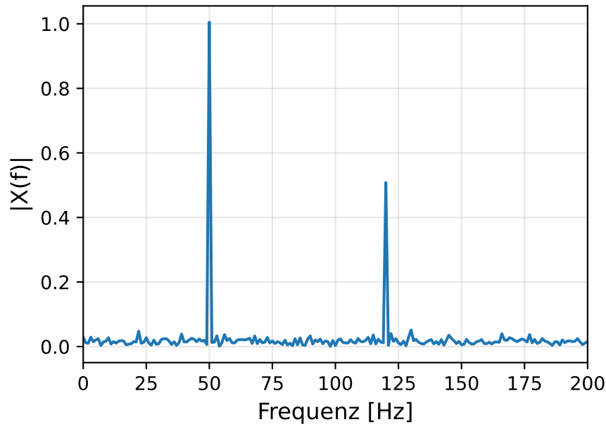
FFT-Spektrum (NumPy)
