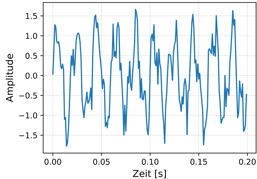
Zeitsignal (Ausschnitt)
