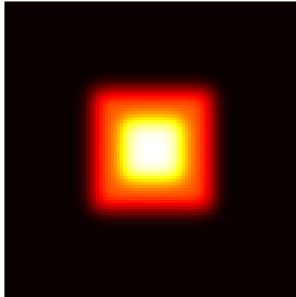
Gauss-Glättung \sigma = 3
