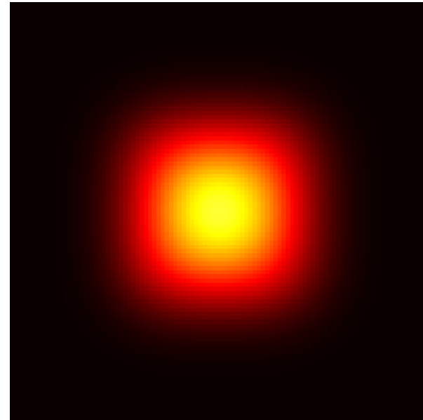
Gauss-Glättung \sigma = 8
