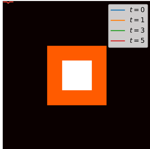
Gauss-Glättung \sigma = 0
