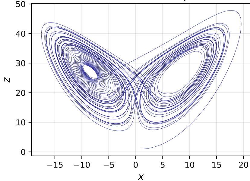
Lorenz-Attraktor (xz-Projektion)
