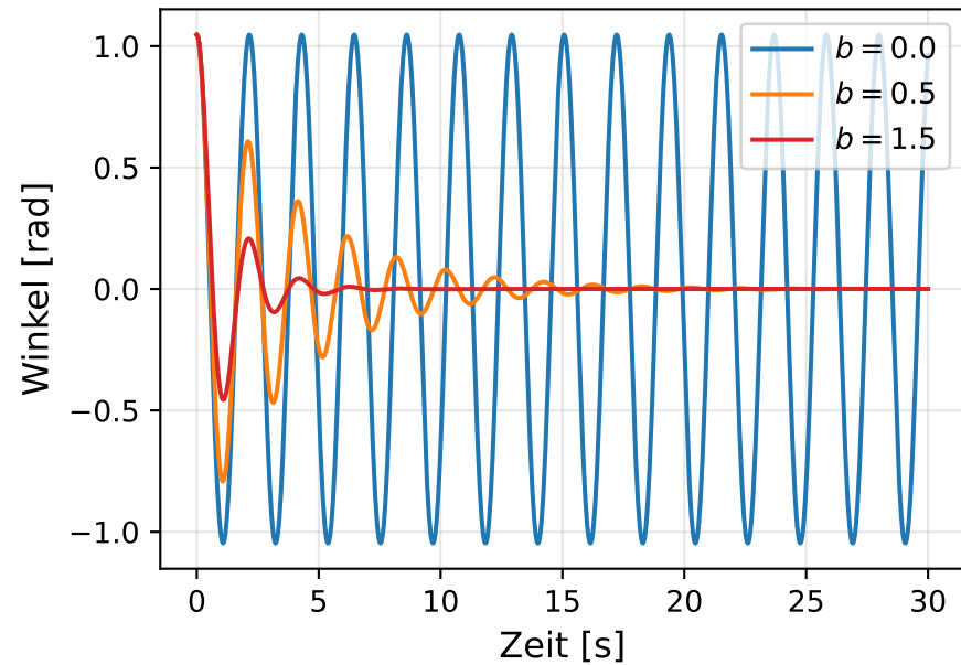
Gedämpftes Pendel
