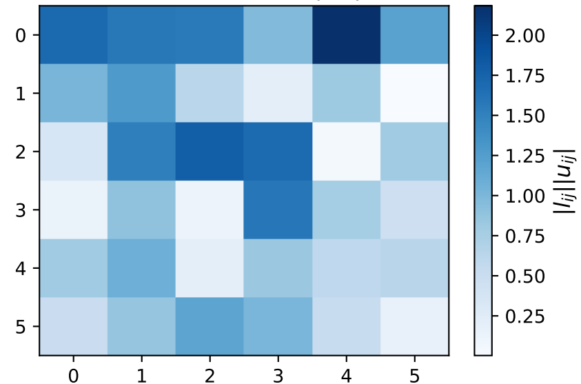
Rekonstruktion |LU|
