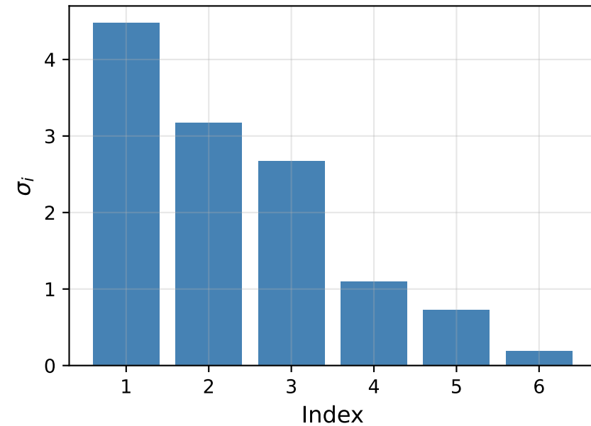
Singuläre Werte (SVD)
