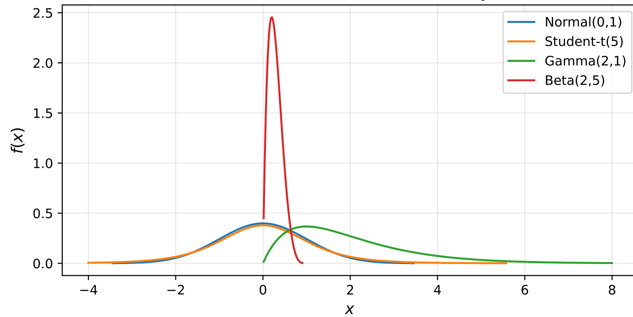
Wahrscheinlichkeitsdichten (SciPy)
