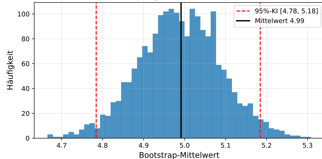
Bootstrap-Konfidenzintervall
