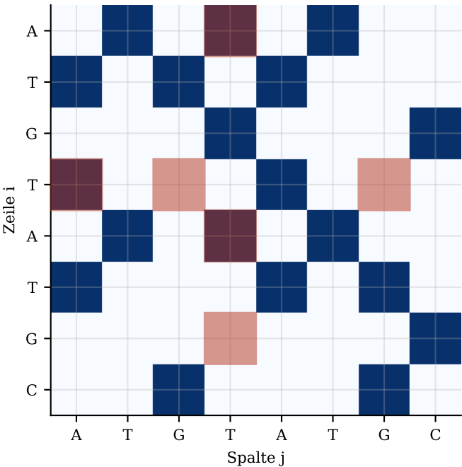
Substitution C→T (Pos. 3) 6 geänderte Einträge (rot)
