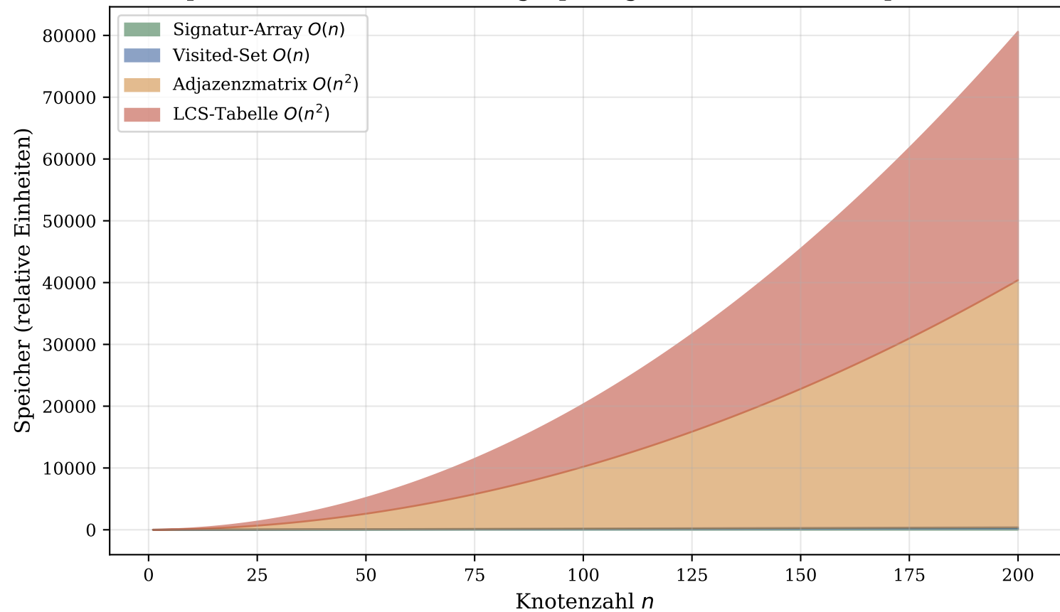
Speicherverbrauch des Subgraph Algorithmus nach Komponenten
