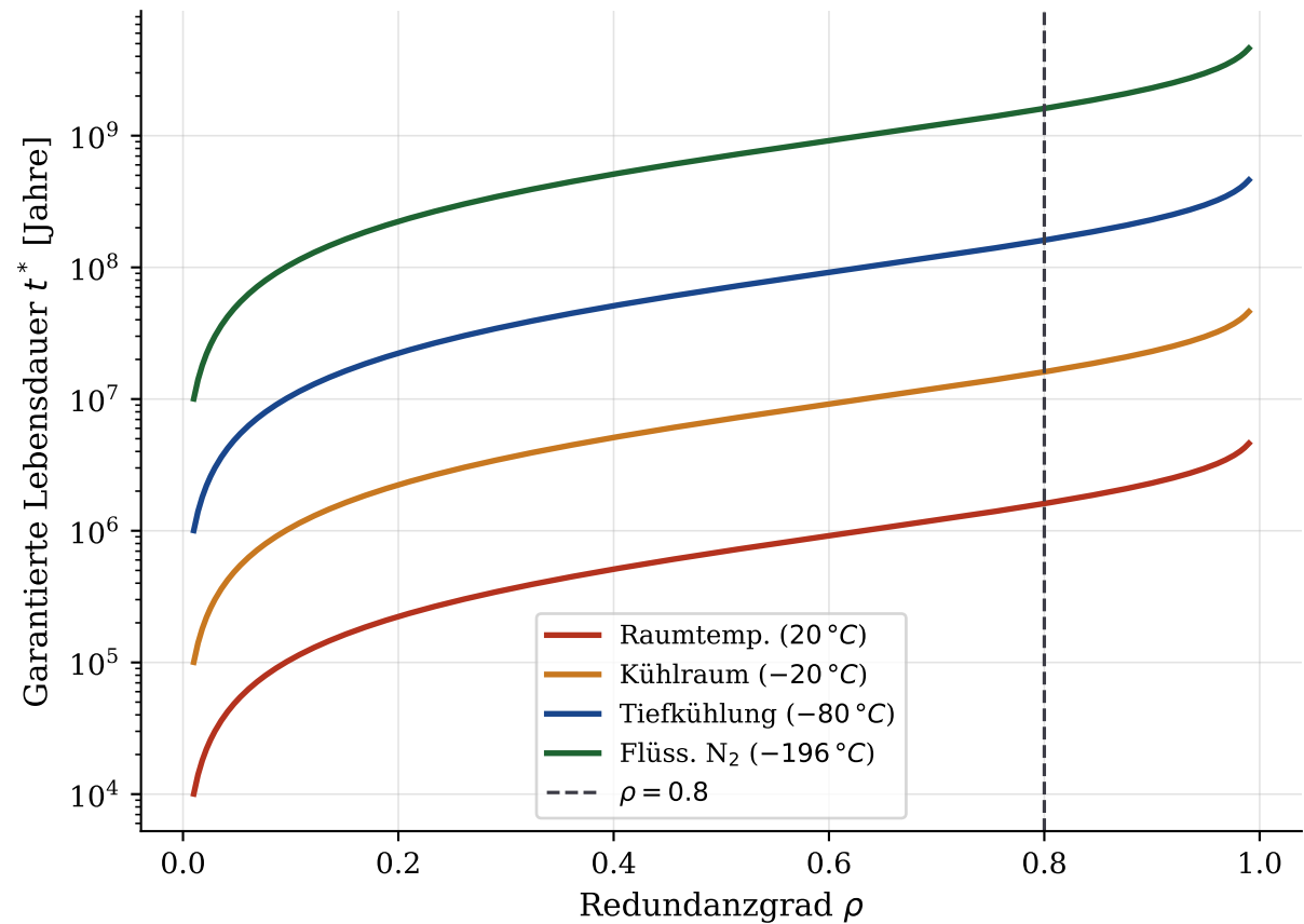
Garantierte Lebensdauer t^* = -\ln(1 - \rho)/\lambda
