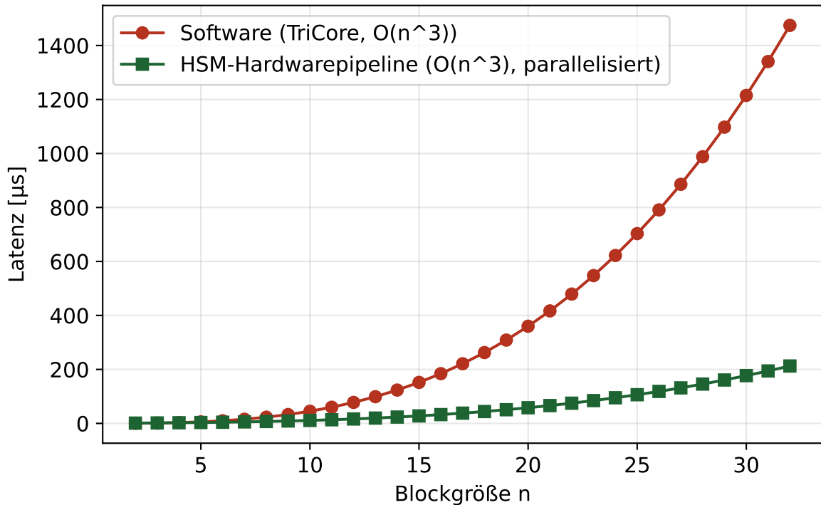
Latenz der Signaturpipeline: Software vs. HSM-Hardware
