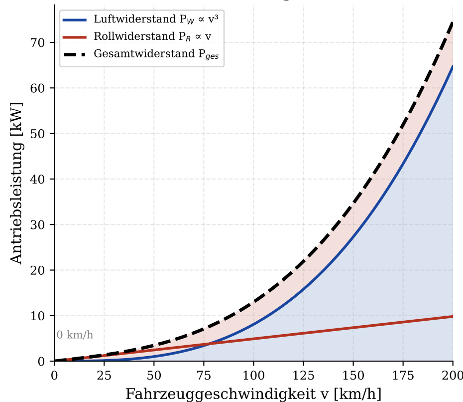
Antriebsleistungsanteile
