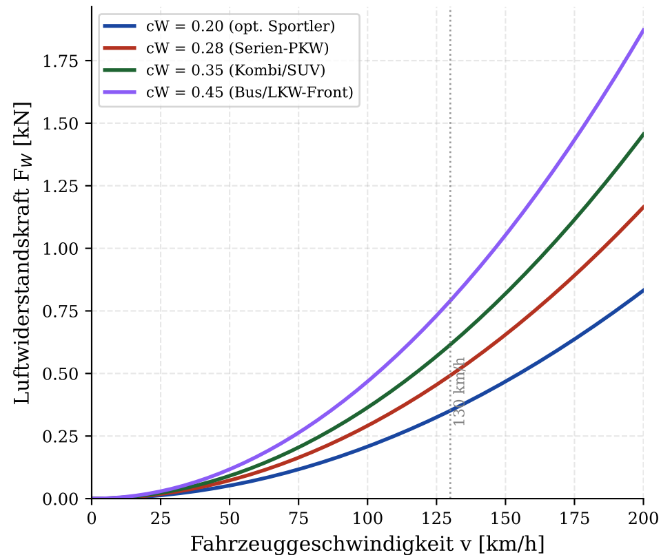
Luftwiderstandskraft
