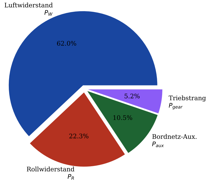
Leistungsverteilung bei 130 km/h (Gesamt: 28.6 kW)
