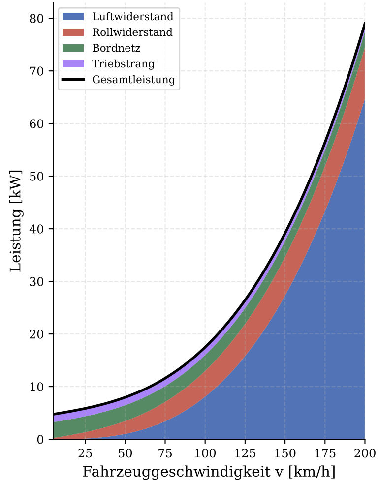
Leistungsanteile über Geschwindigkeit
