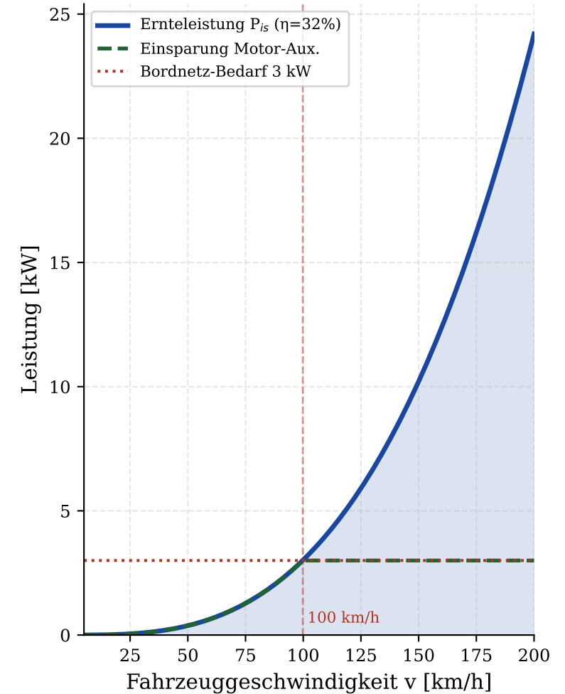
Netto-Energiegewinn der Hilfsverbraucher
