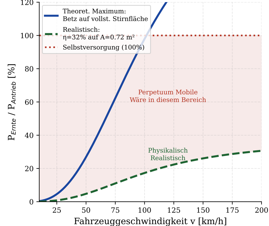
Grenzen der Selbstversorgung: Warum kein Perpetuum Mobile möglich ist
