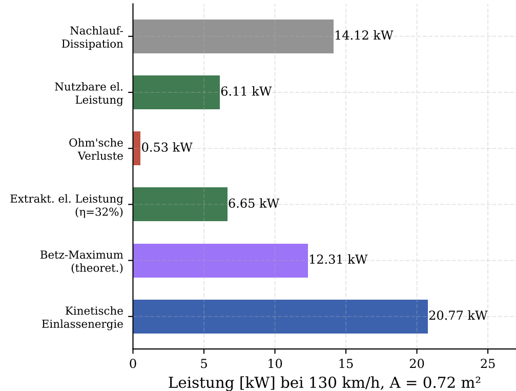
Energiefluss-Bilanz (Sankey-Näherung)
