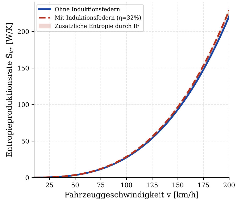
Entropieproduktion mit und ohne Induktionsfedern
