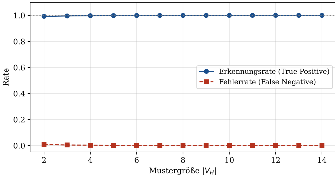
Erkennungsrate des Subgraph Algorithmus im JCL
